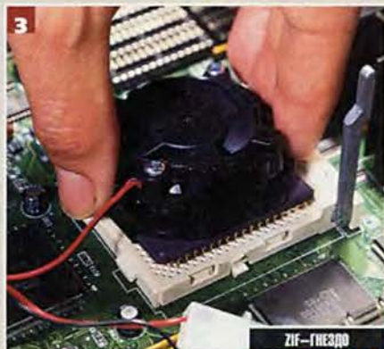
ZIF-ГНЕЗДО
