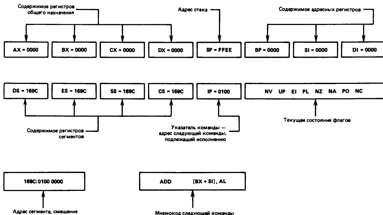
Схема начального вывода программы Debug
