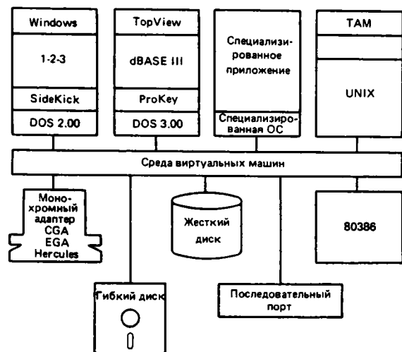
Рис. А. Работа под управлением программы VM/386 фирмы Softquad Systems, каждая виртуальная машина имеет собственную операционную систему и текущую задачу. Каждая действует так, как будто она монополюно владеет процессором
