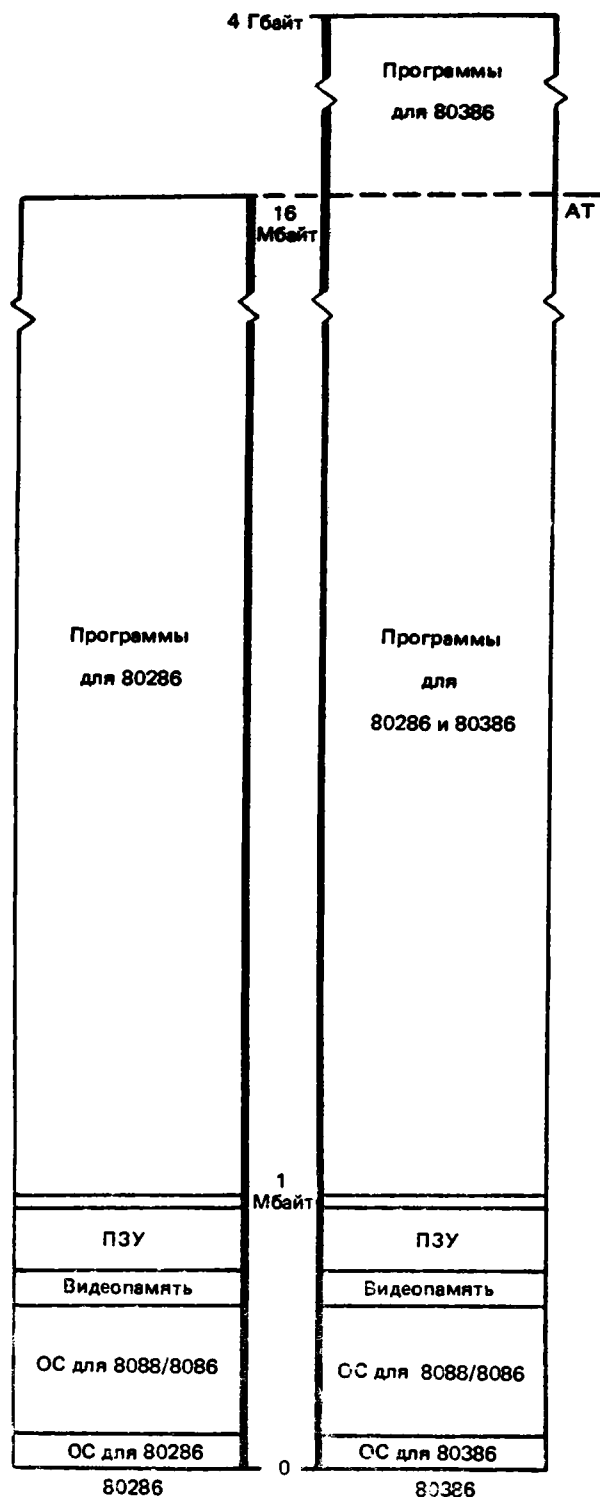
Модели работы микропроцессоров 80286 и 80386 в защищенном режиме
