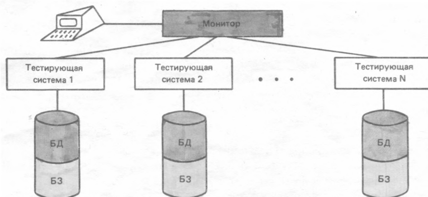
Рис. 3. Структура формирования "батарей" тестов ПДС
