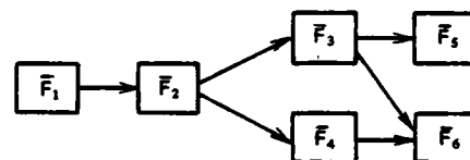
Рис. 6. Параллельная структура обработки
