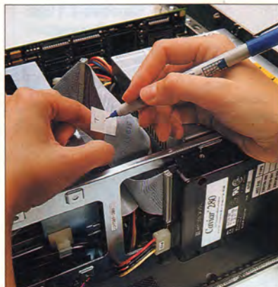
Пометьте, как подключены плоские серые кабели к разным дисководам.
