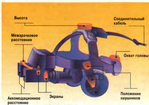
Основные элементы конструкции и регулировки шлема
