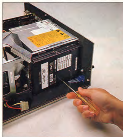
Закрепите новый жесткий диск винтами в отсеке.
