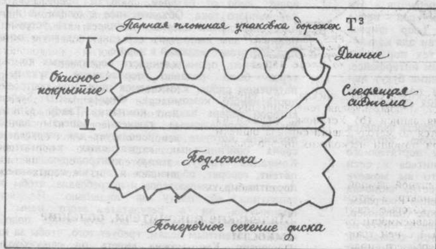
Рис. 4. Сервосистема T3 фирмы Brier (Twin Tier Tracking) использует два слоя магнитной информации. Более глубокий слой является постоянным и обеспечивает информацию о дорожке.
