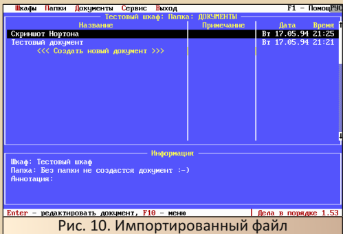
Рис. 10. Импортированный файл
