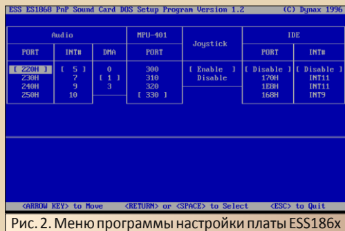
Рис. 2. Меню программы настройки платы ESS186x
