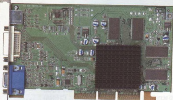
ATI Radeon 7000.
