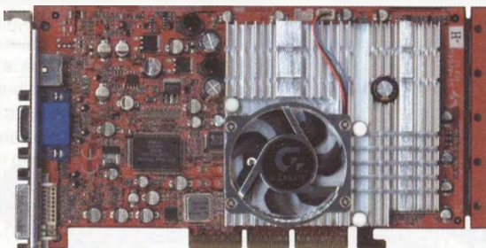
Gigabyte MAYA AP64S-H Radeon 7500 Pro.
