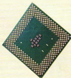
INTEL CELERON 1300
