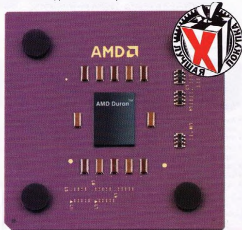
AMD Duron 1200.
