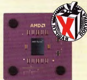
AMD DURON 1200
