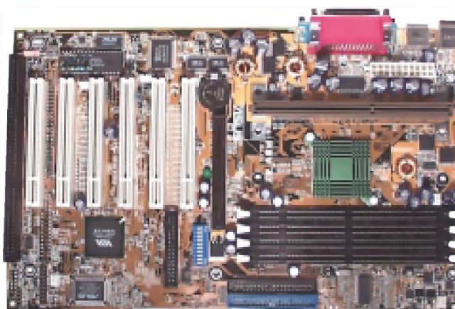
ASUS P3V4X
