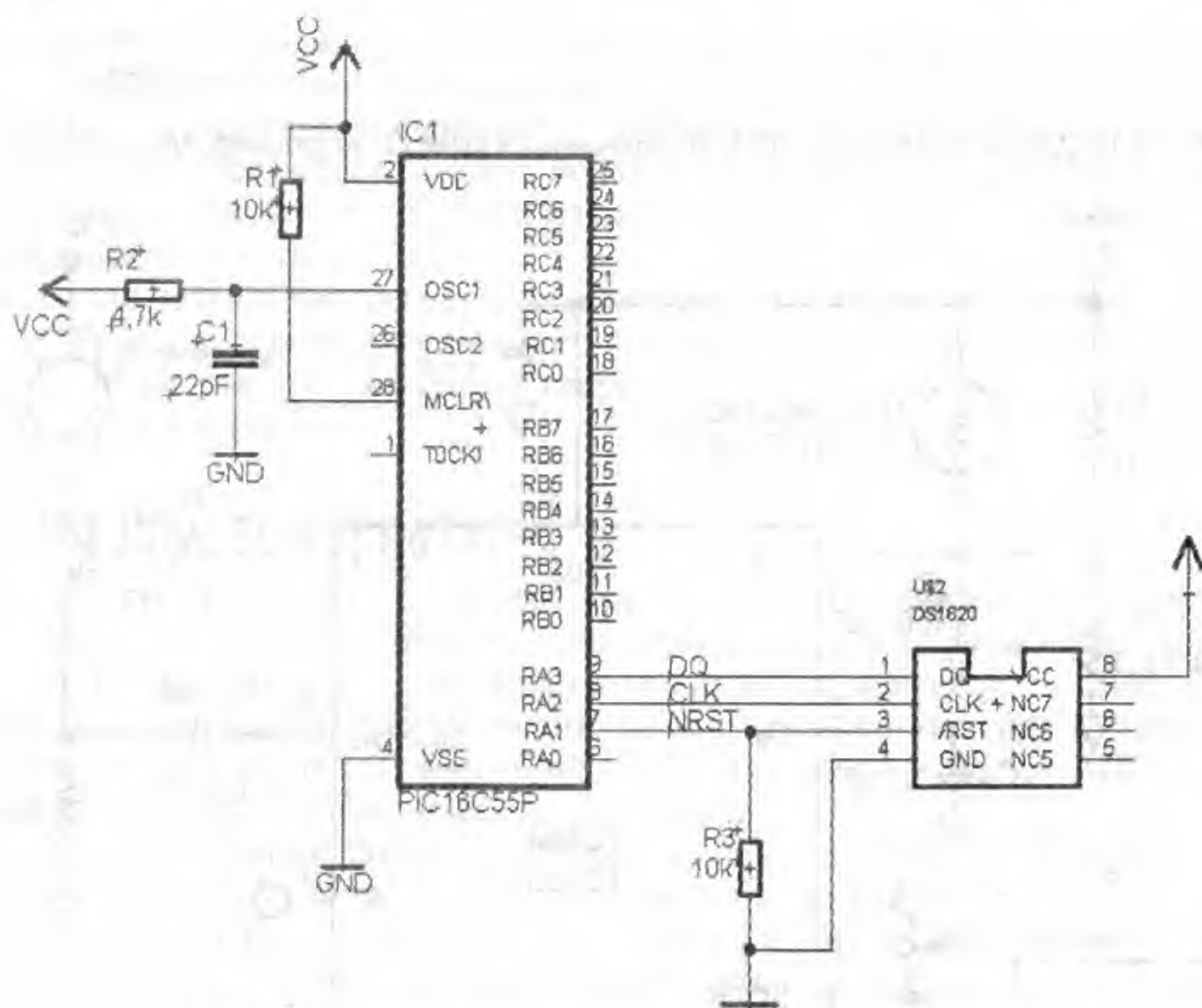
Рис. 11.21. Пример включения цифрового термометра DS1620
