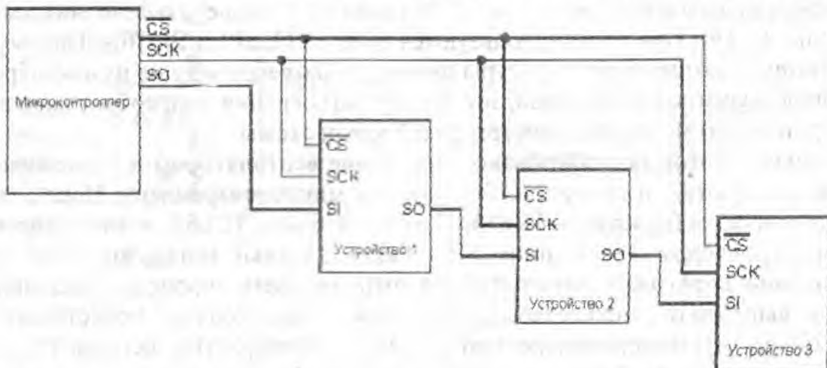
Рис. 11.18. Гирляндное подключение нескольких цифровых потенциометров
