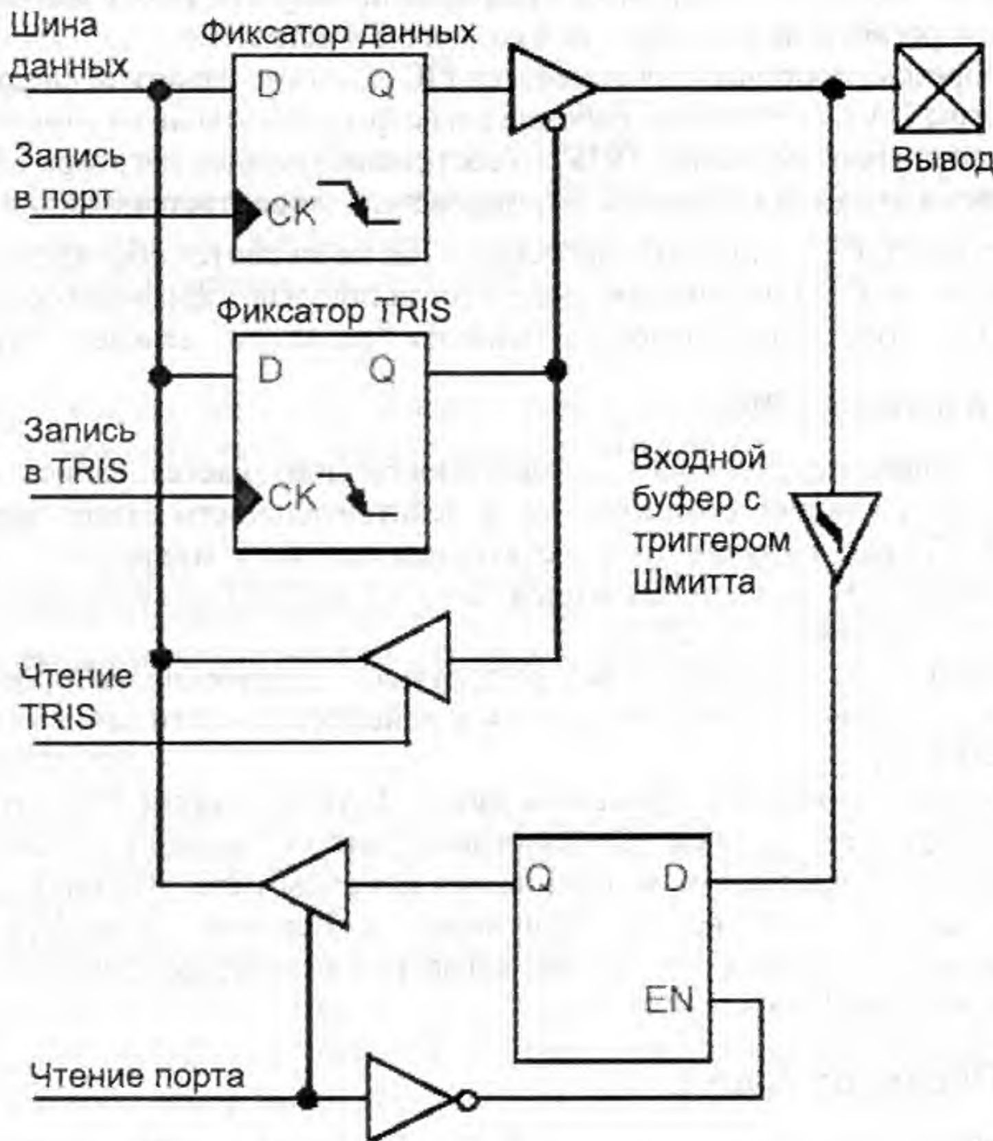
Рис. 3.1. Типичный порт
