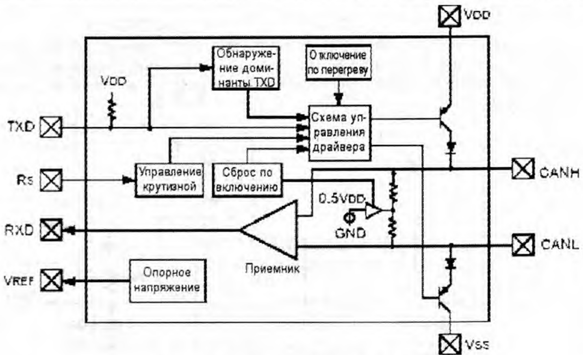
Рис. 11.3. Преобразователь уровня MCP2551
