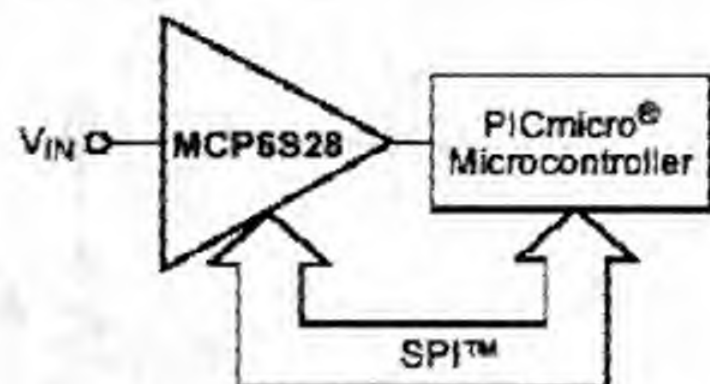
Рис. 11.13. Пример использования PGA с микроконтроллером PIC
