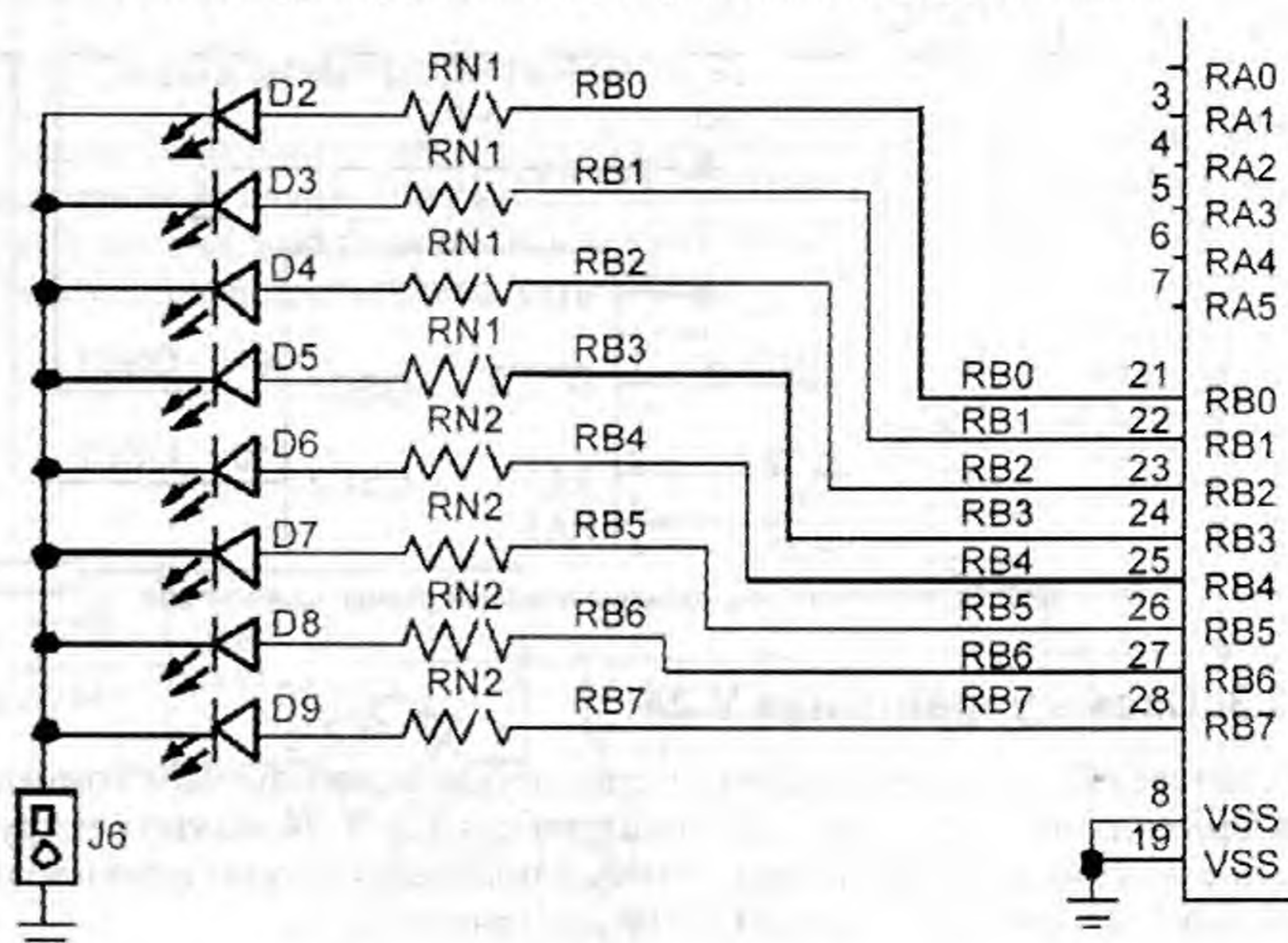
Рис. 10.4. Светодиоды с добавочными резисторами
