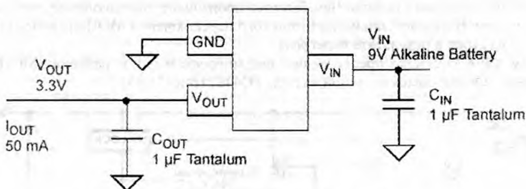
Рис. 11.23. Питание 3,3 В в устройстве на 9 В
