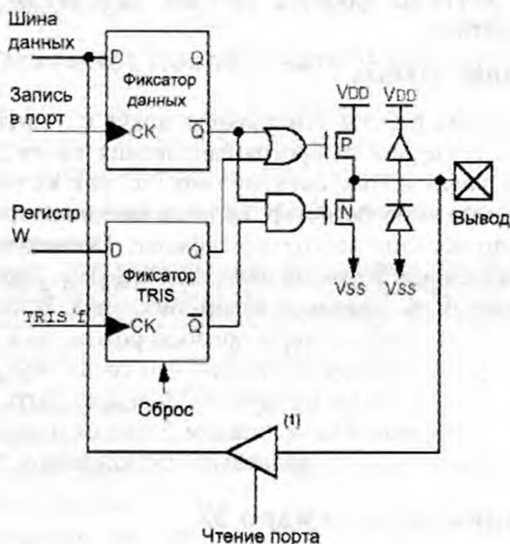
Рис. 5.2. Блок-схема вывода порта
