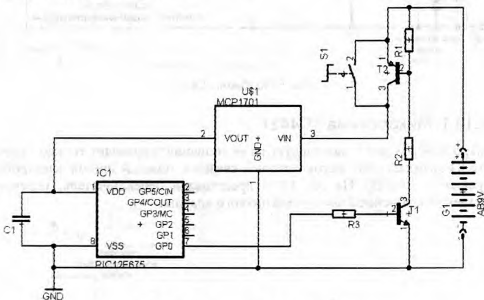
Рис. 11.24. Отключение батареи 9 В
