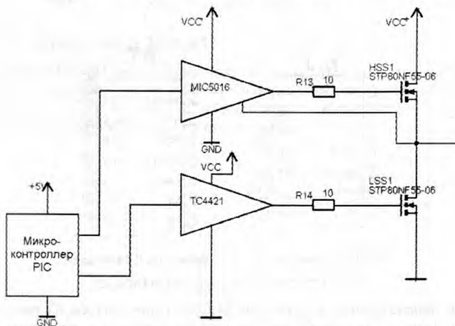
Рис. 11.29. Полумостовая схема с переключателями MIC5016 и TC4421
