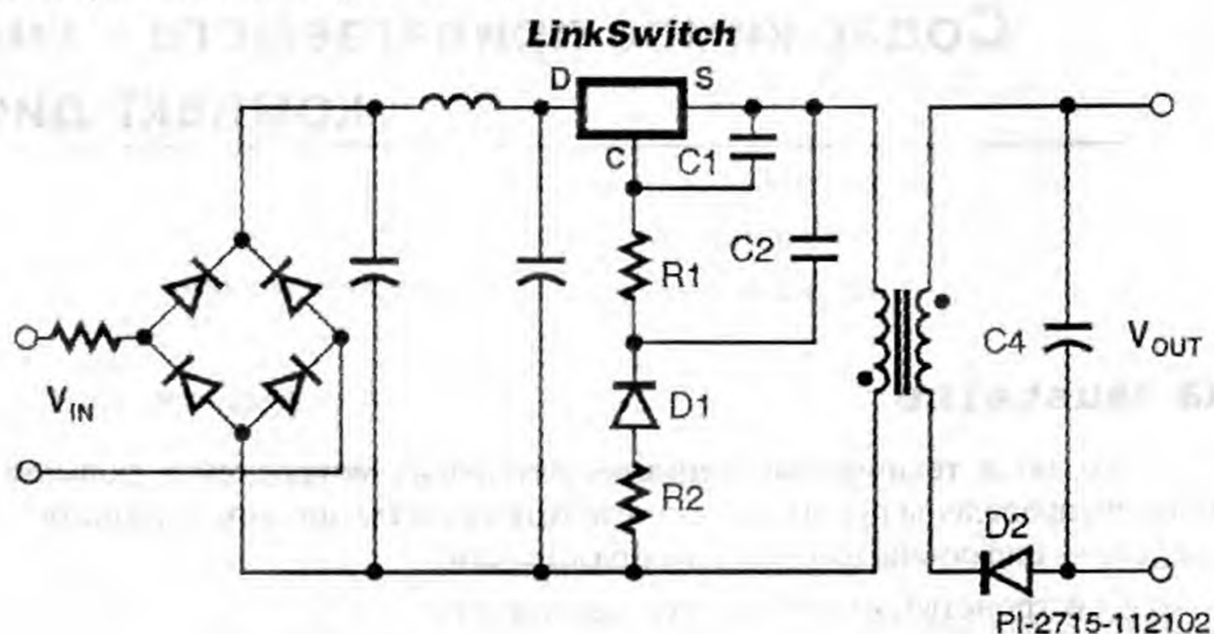
Рис. 11.32. Пример схемы с применением LNK500
