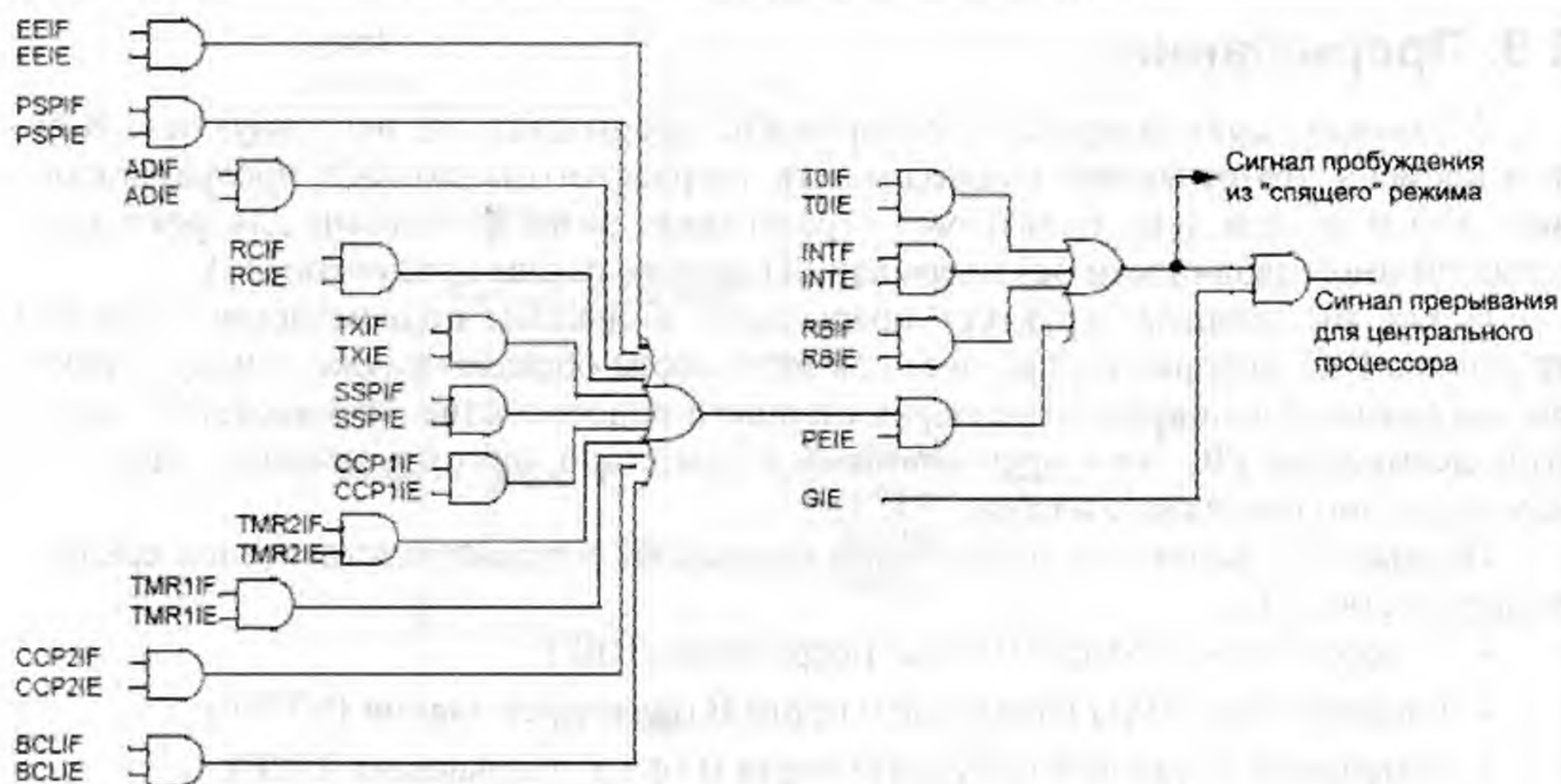
Рис. 1.3. Пример структуры прерываний
