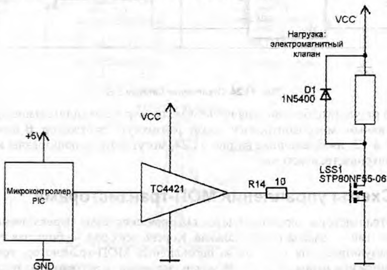
Рис. 11.26. Пример применения микросхемы TC4421
