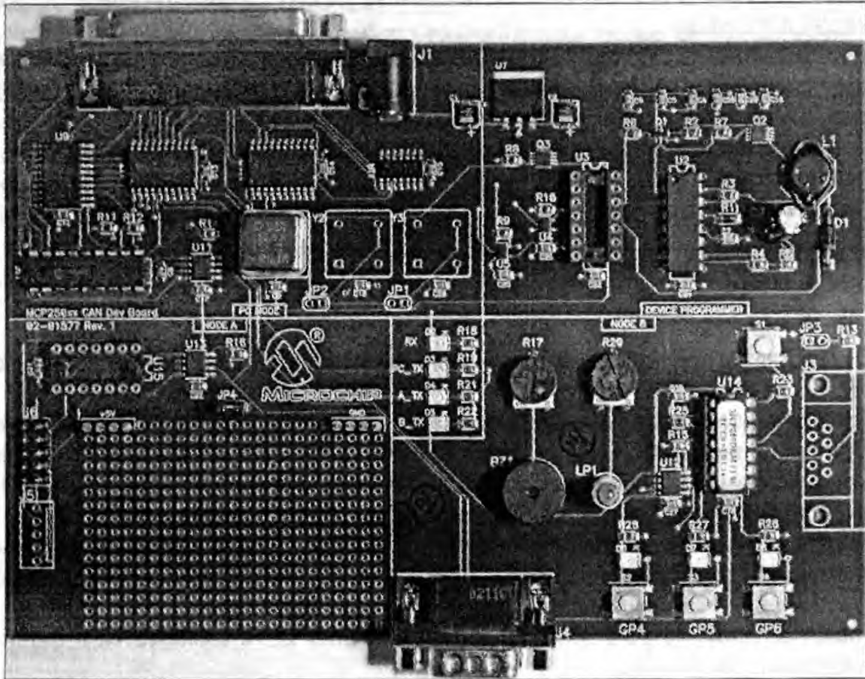
Рис. 10.19. Демо-плата MCP250XX
