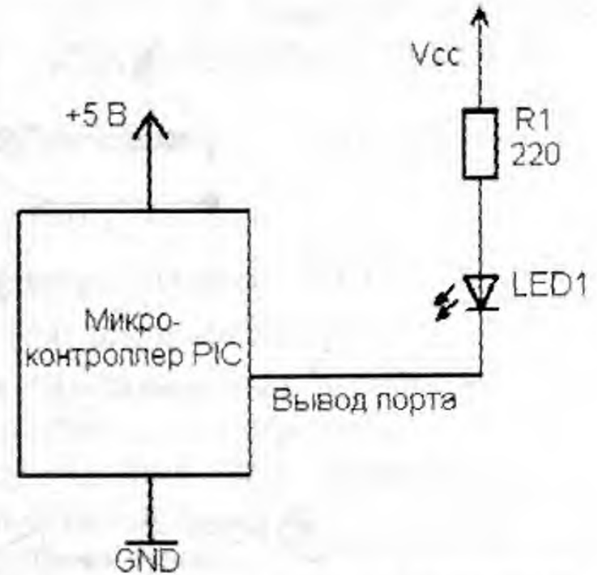
Рис. 1.1. Нагрузка вывода светодиодом
