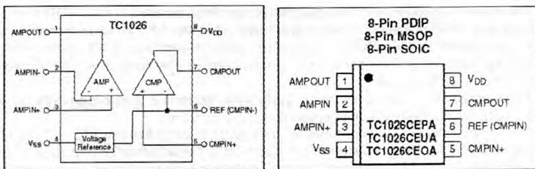
Рис. 11.14. Небольшой линейный блок
