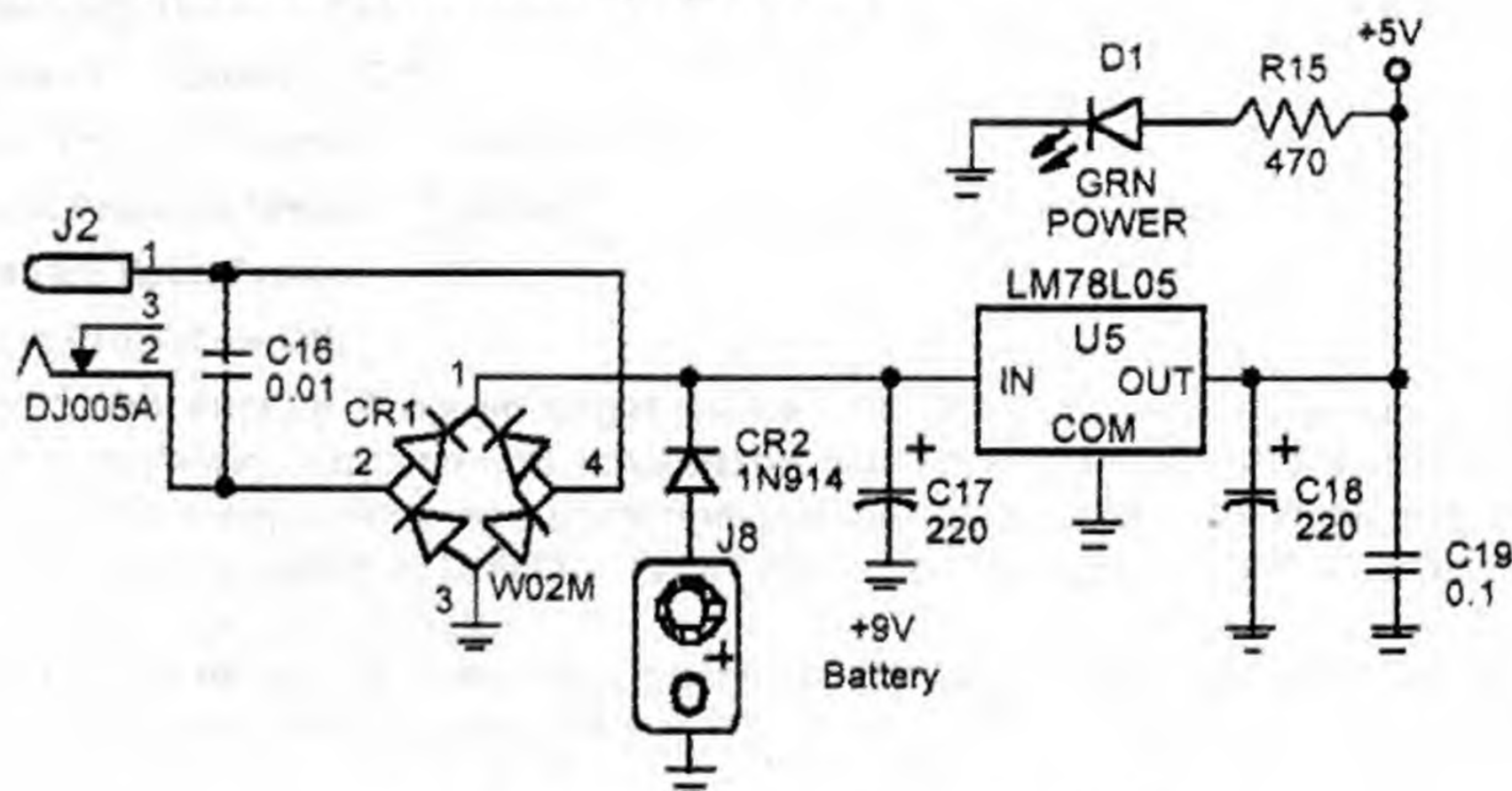
Рис. 10.1. Типичная схема питания демо-платы
