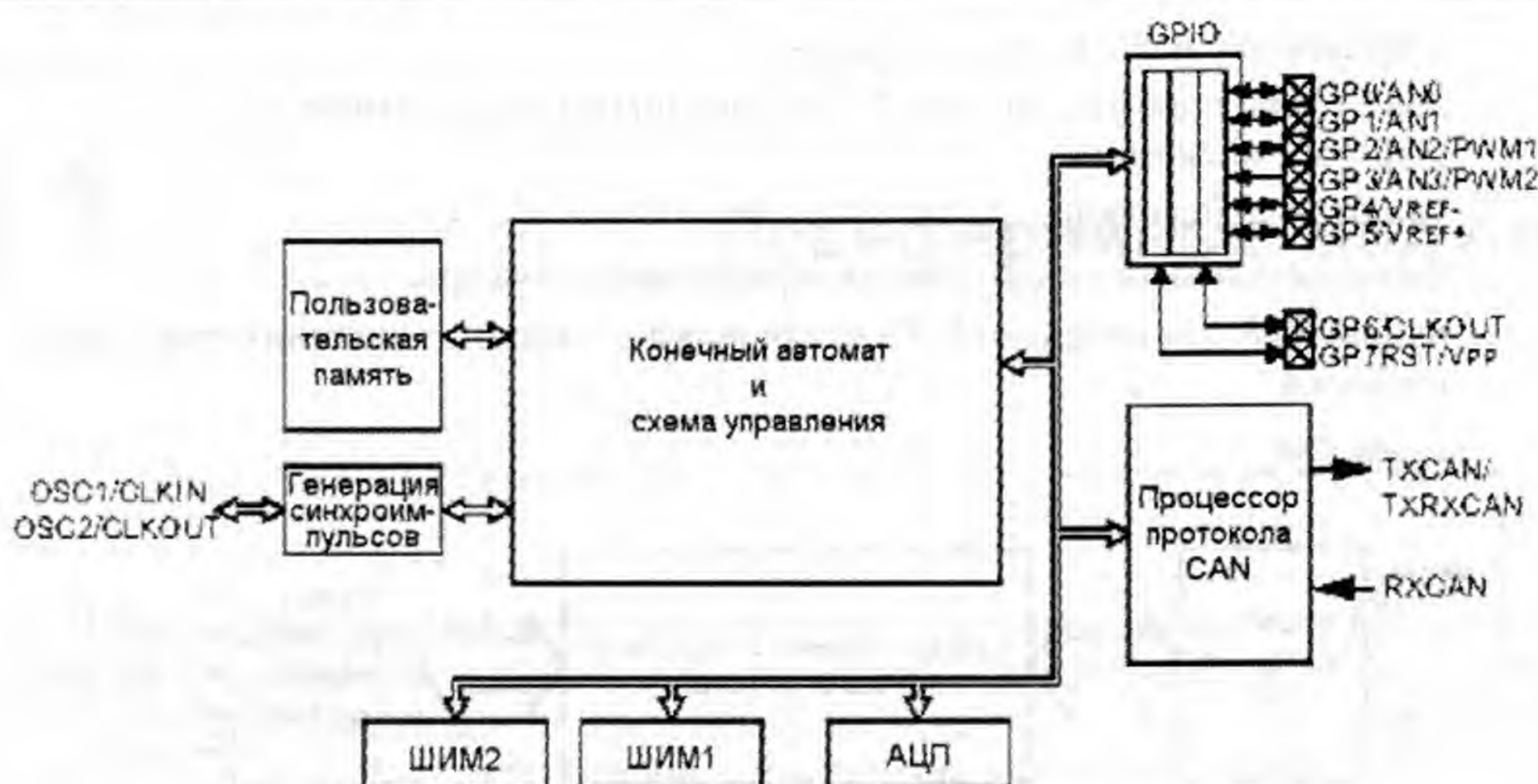
Рис. 11.2. Интерфейс CAN обходится без микроконтроллера PIC
