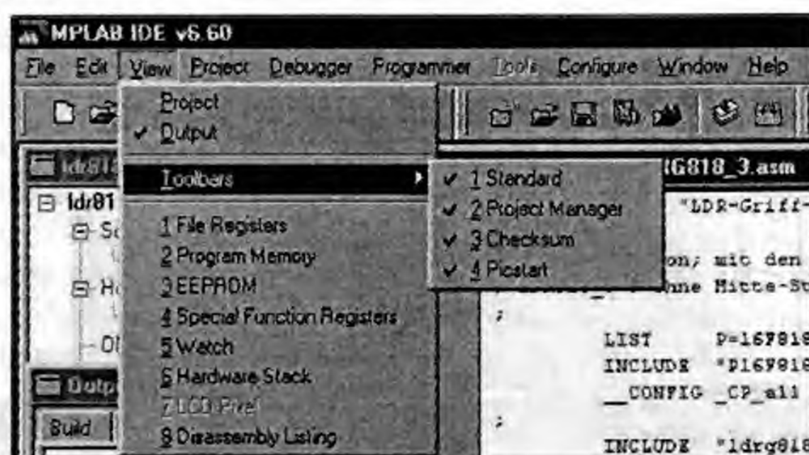
Рис. 8.7. Меню View
