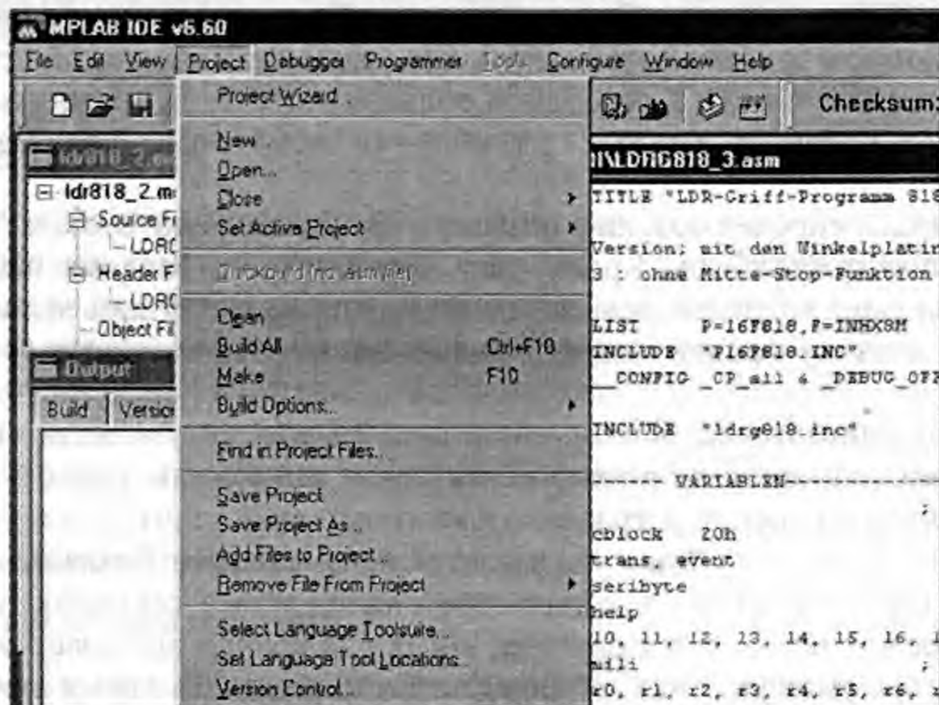
Рис. 8.14. Меню Project
