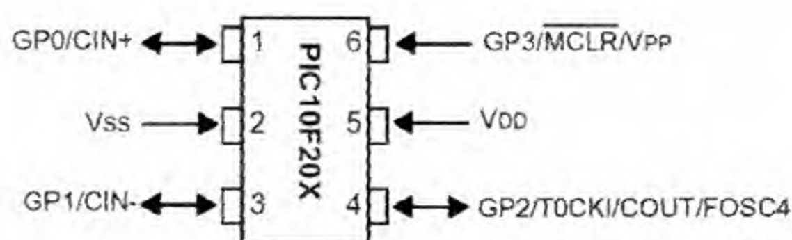
Рис. 5.1. Малейший из PIC
