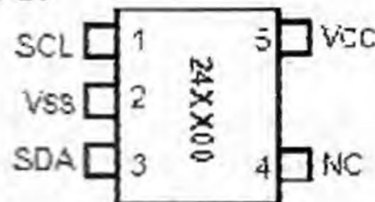
Рис. 11.8. Миникорпуса микросхемы 24LC00
