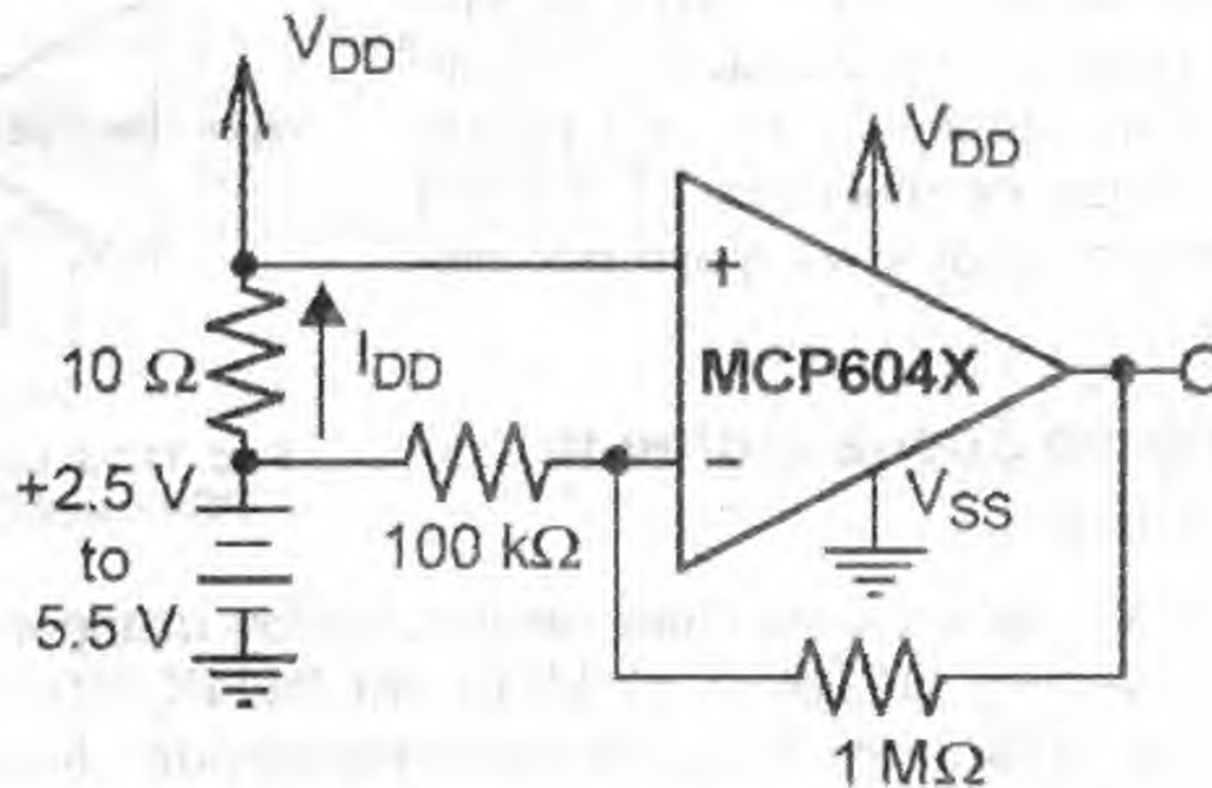
Рис. 11.11. Пример применения ОУ MCP604X
