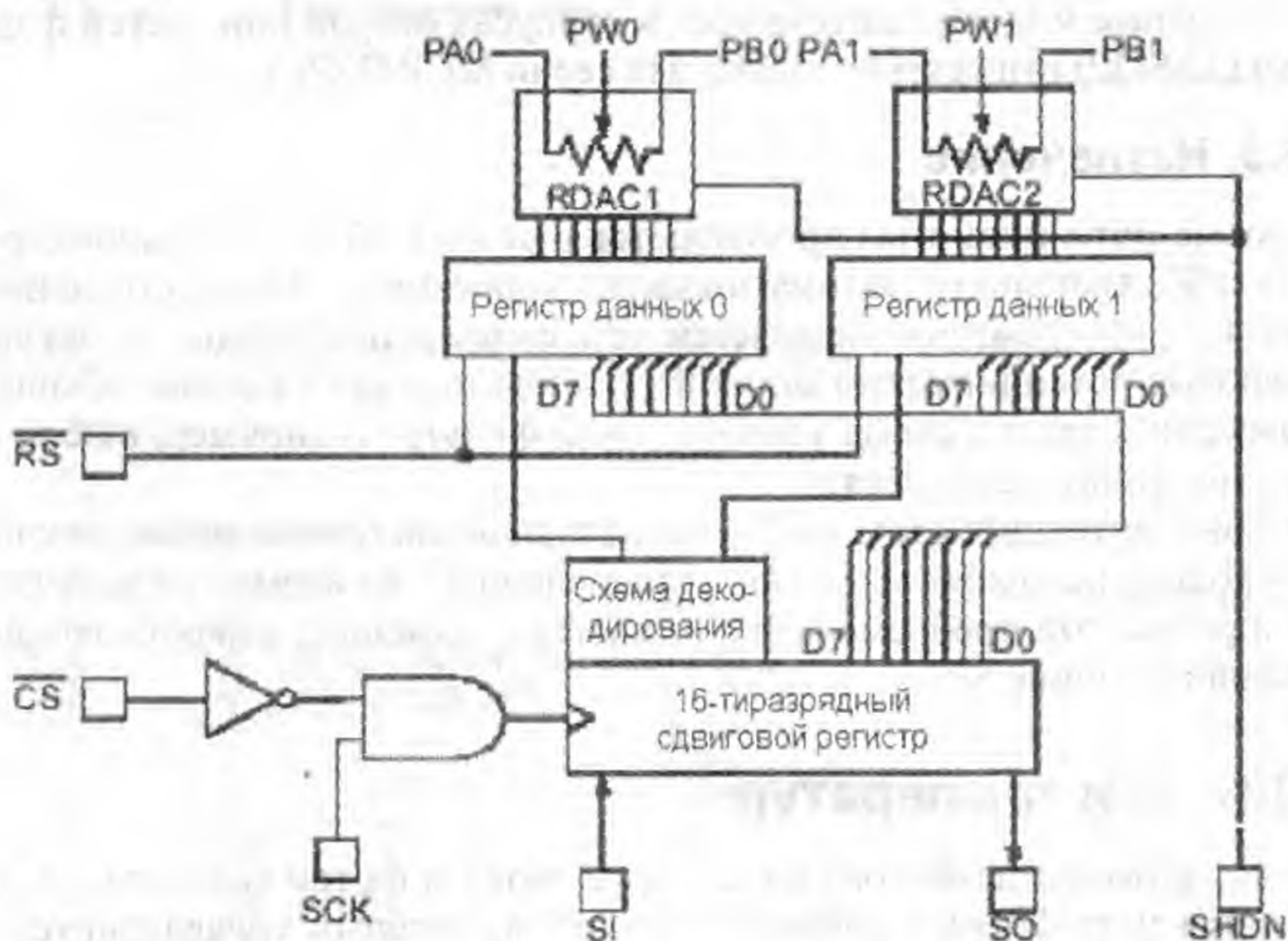
Рис. 11.17. Схема цифрового потенциометра MCP42XXX
