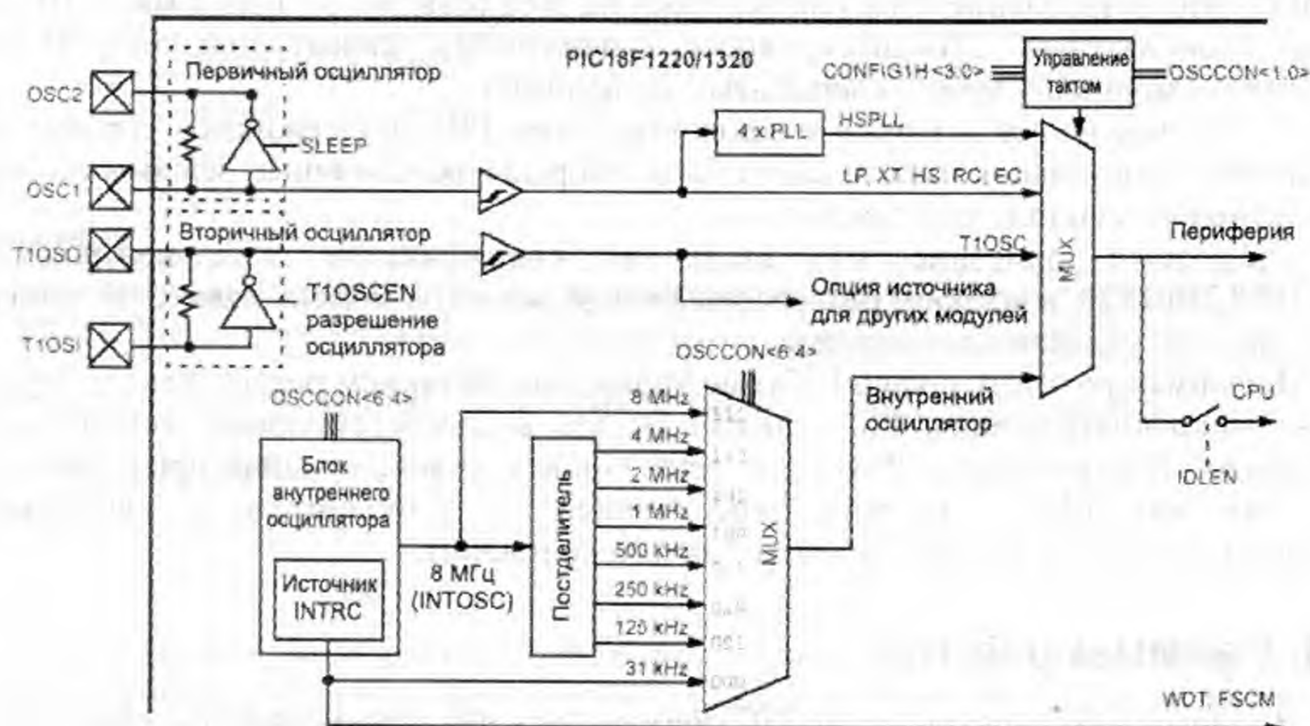
Рис. 4.1. Формирование тактовых импульсов в микроконтроллере 18F1220
