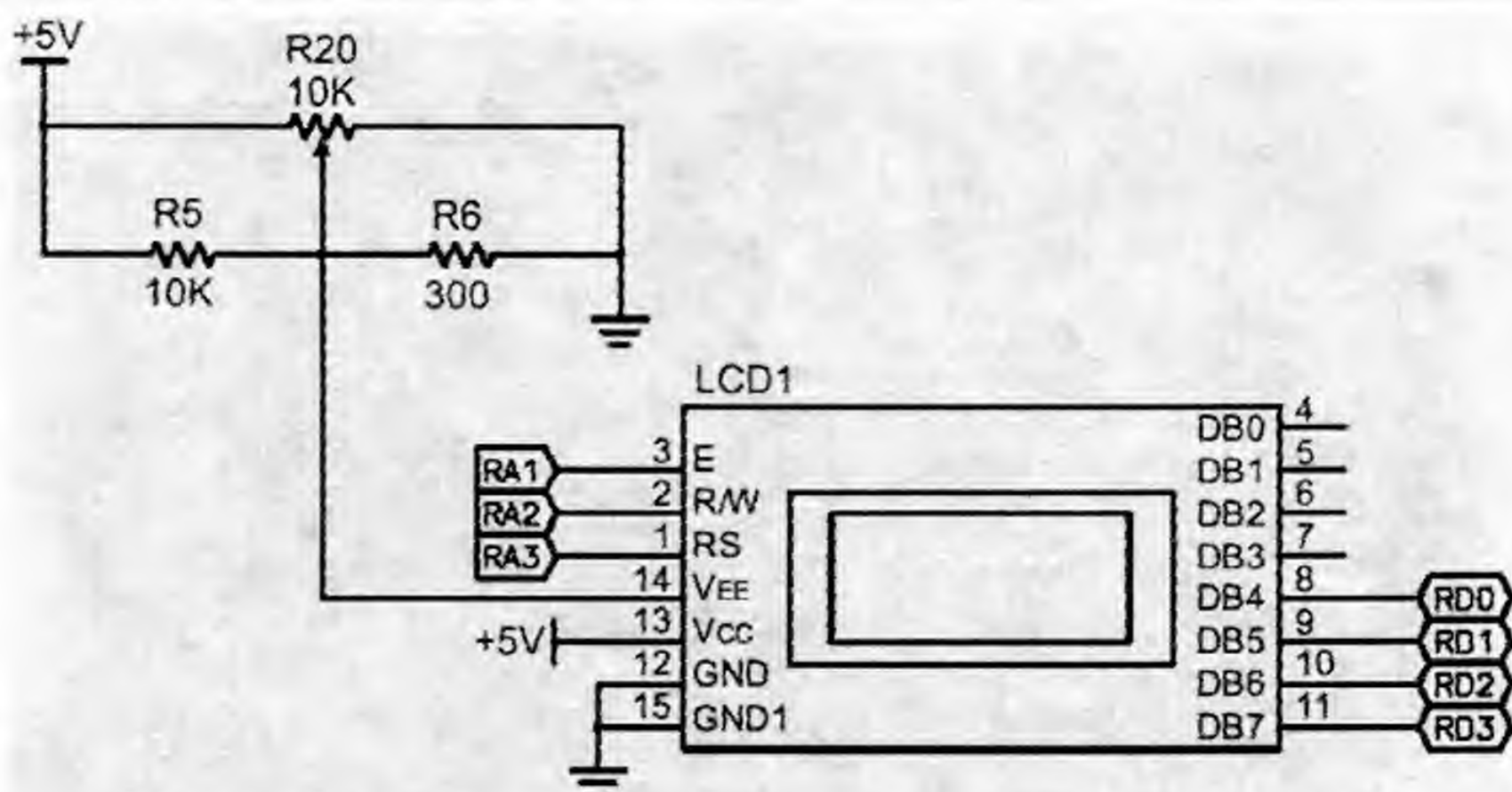
Рис. 10.8. ЖК-дисплей с контроллером и четырехразрядной шиной данных
