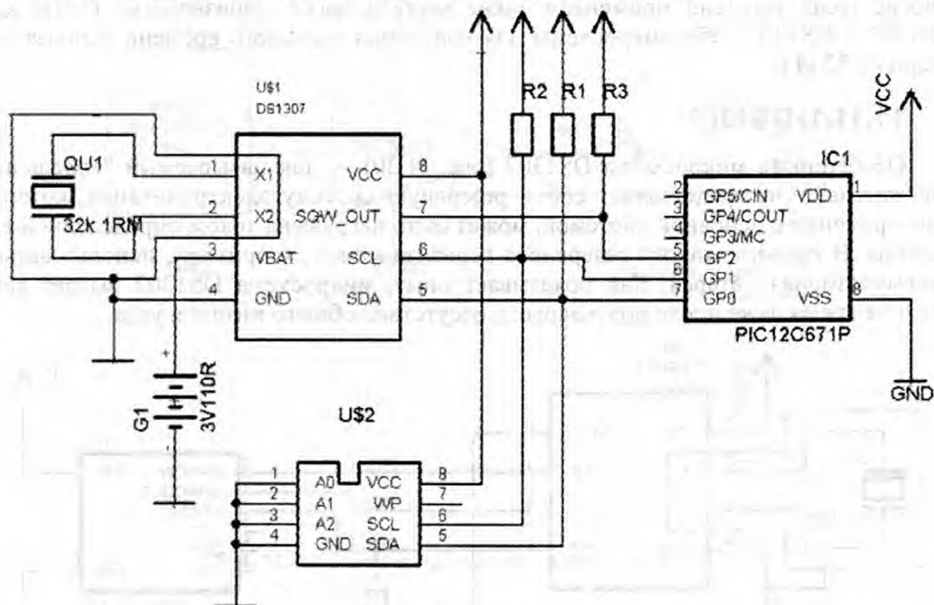
Рис. 11.31. Модуль DS1307 в качестве часов реального времени
