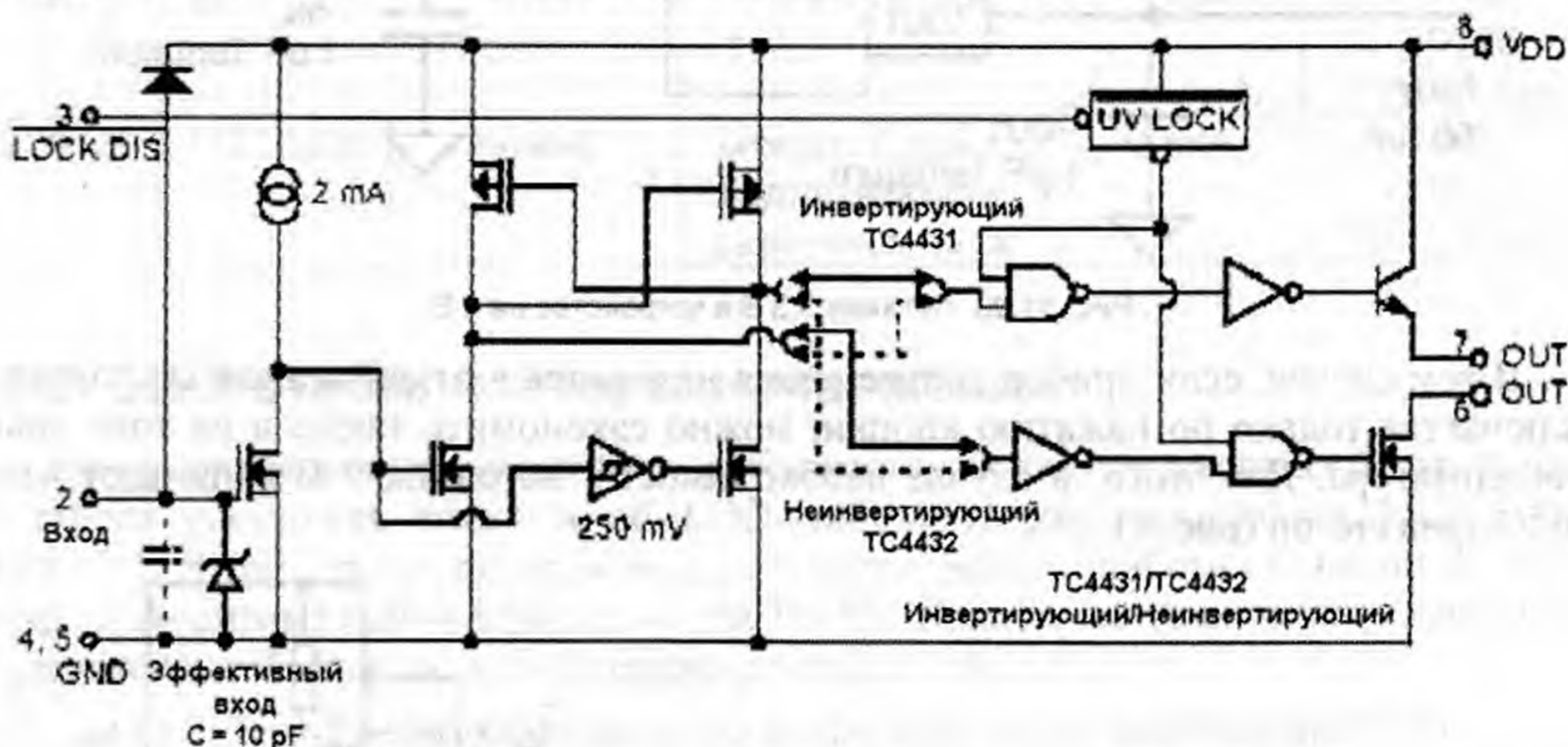
Рис. 11.25. Схема TC4421
