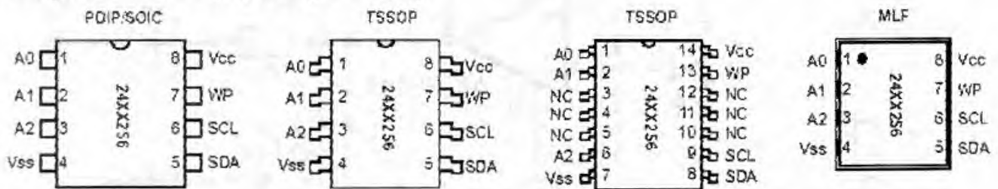
Рис. 11.7. Различные типы корпусов для микросхем EEPROM с интерфейсом I 2 C
