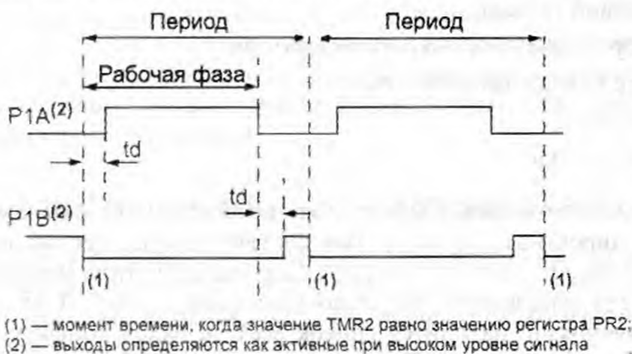
Рис. 1.5. Задержка мертвой зоны
