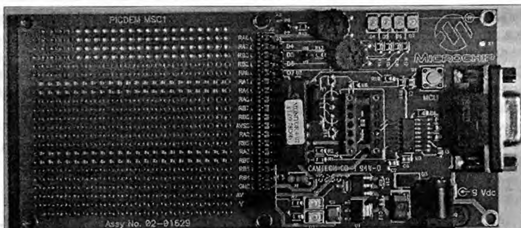
Рис. 10.16. Демо-плата PICDEM MSC
