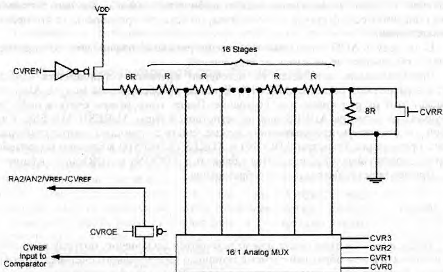
Рис. 1.4. Модуль опорного напряжения
