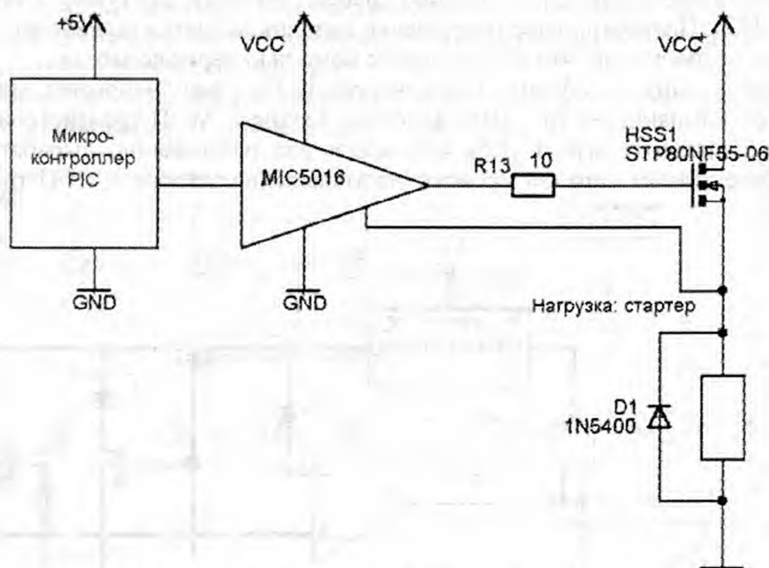
Рис. 11.28. Пример использования микросхемы MIC5016
