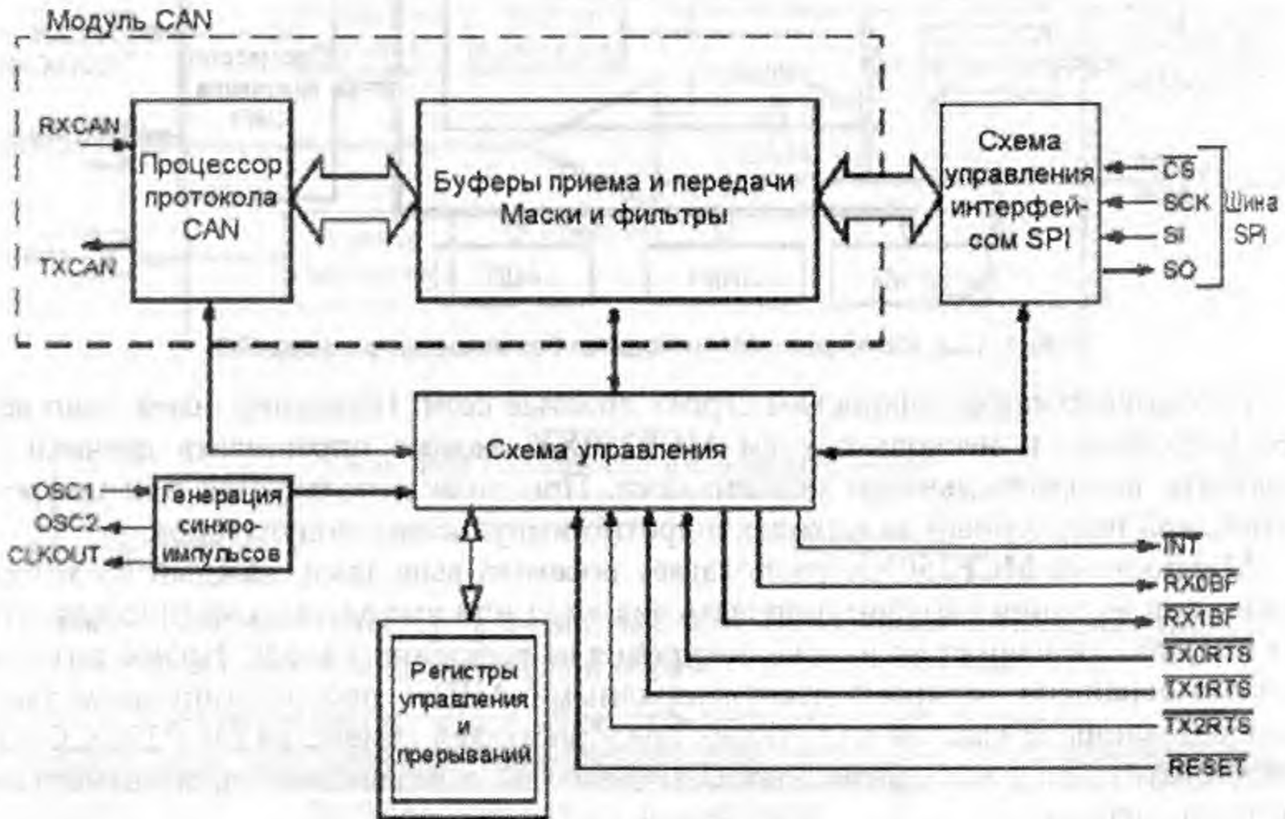
Рис. 11.1. Завершенный CAN-контроллер с шиной SPI
