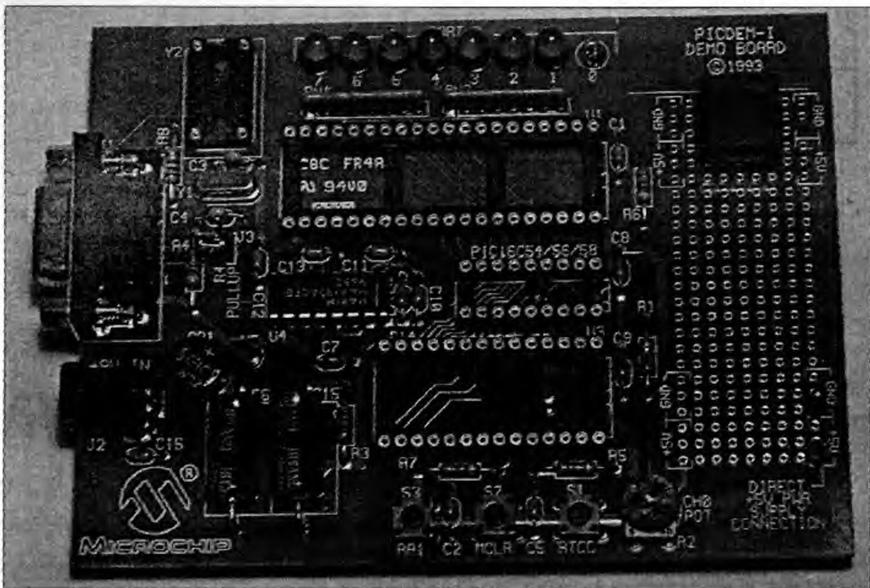
Рис. 10.6. Плата PICDEM1 для семейства 5X и 40-выводных представителей семейства 17
