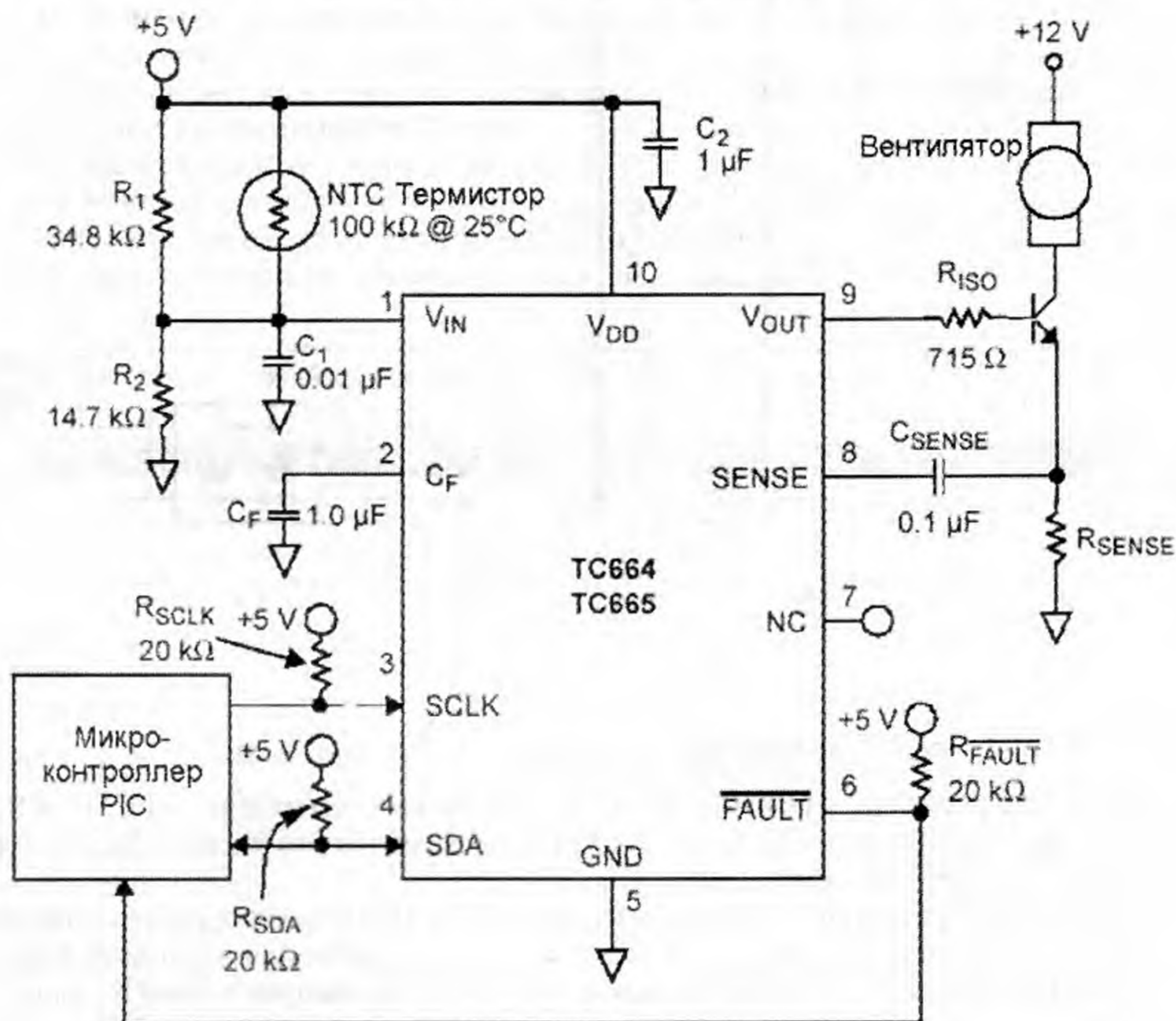
Рис. 11.20. Типичное применение микросхемы TC664
