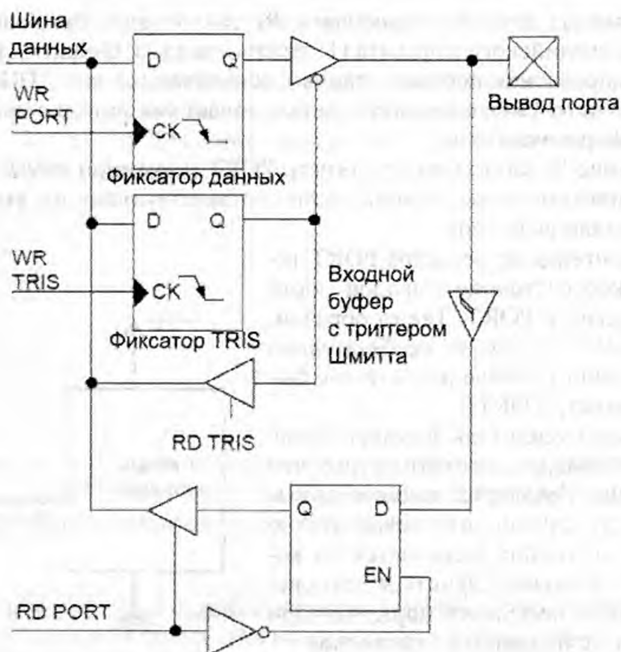
Рис. 1.2. Типичный порт ввода-вывода
