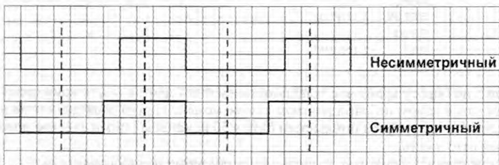
Рис. 2.4. Несимметричность сигналов LIN
