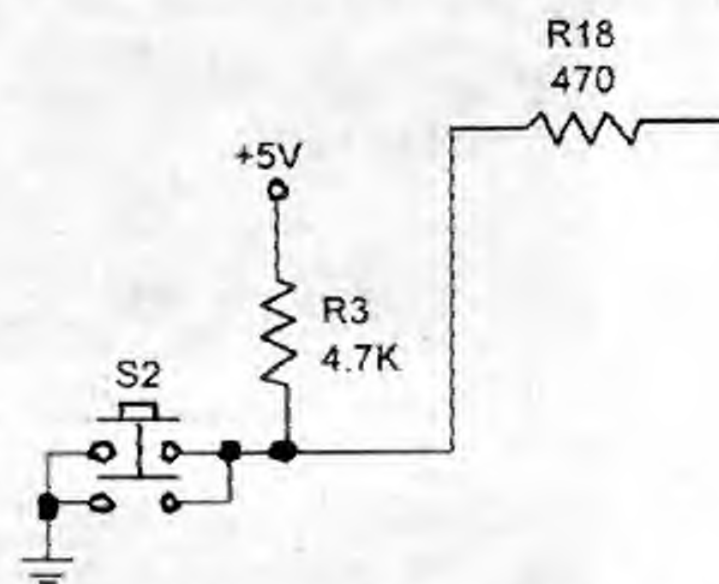
Рис. 10.5. Типичная кнопка демо-платы
