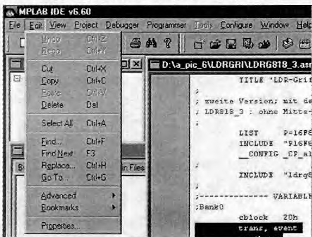
Рис. 8.4. Меню Edit
