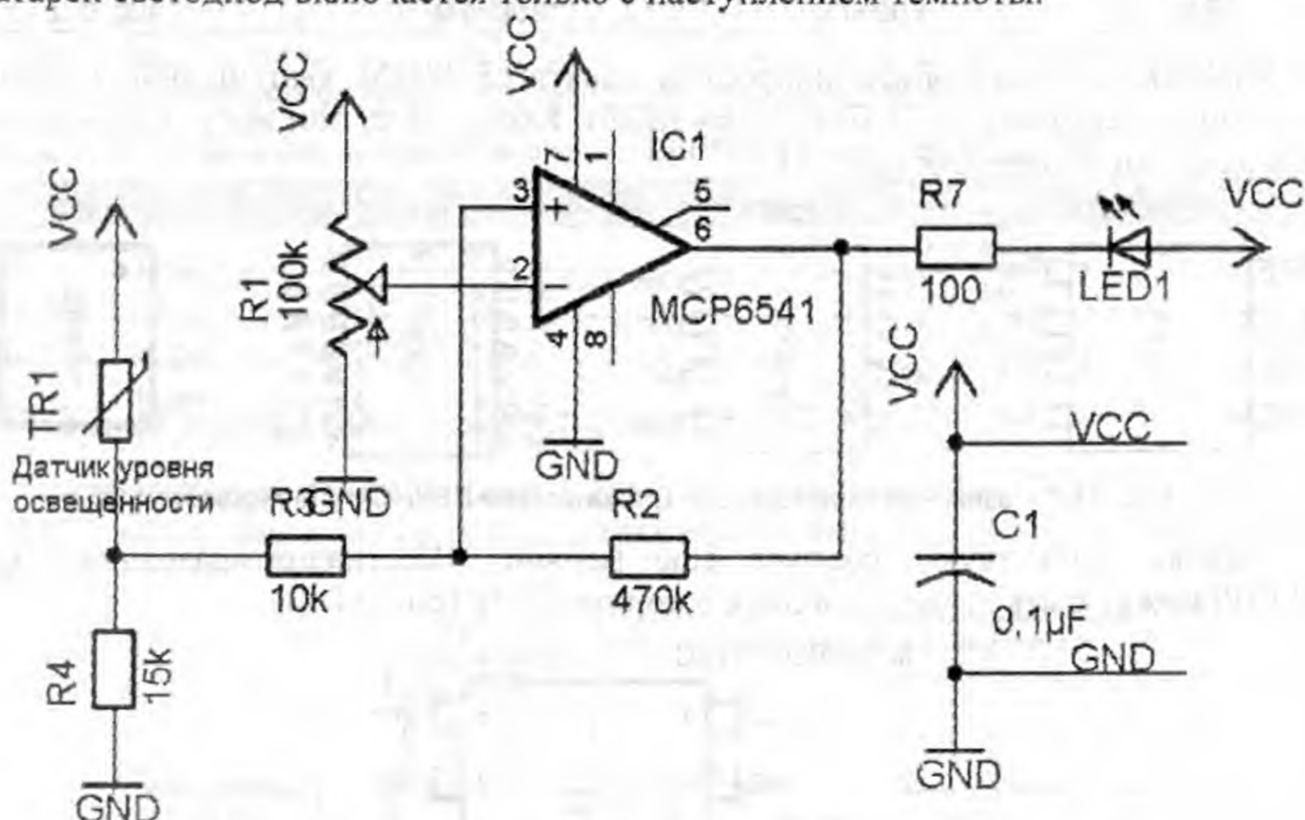
Рис. 11.9. Схема автоматической "свечки"
