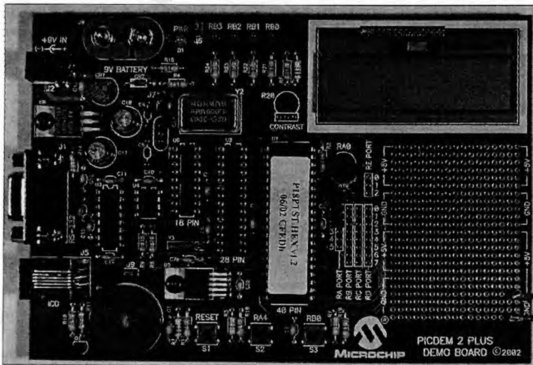
Рис. 10.7. Плата PICDEM2 plus с ЖК-дисплеем
