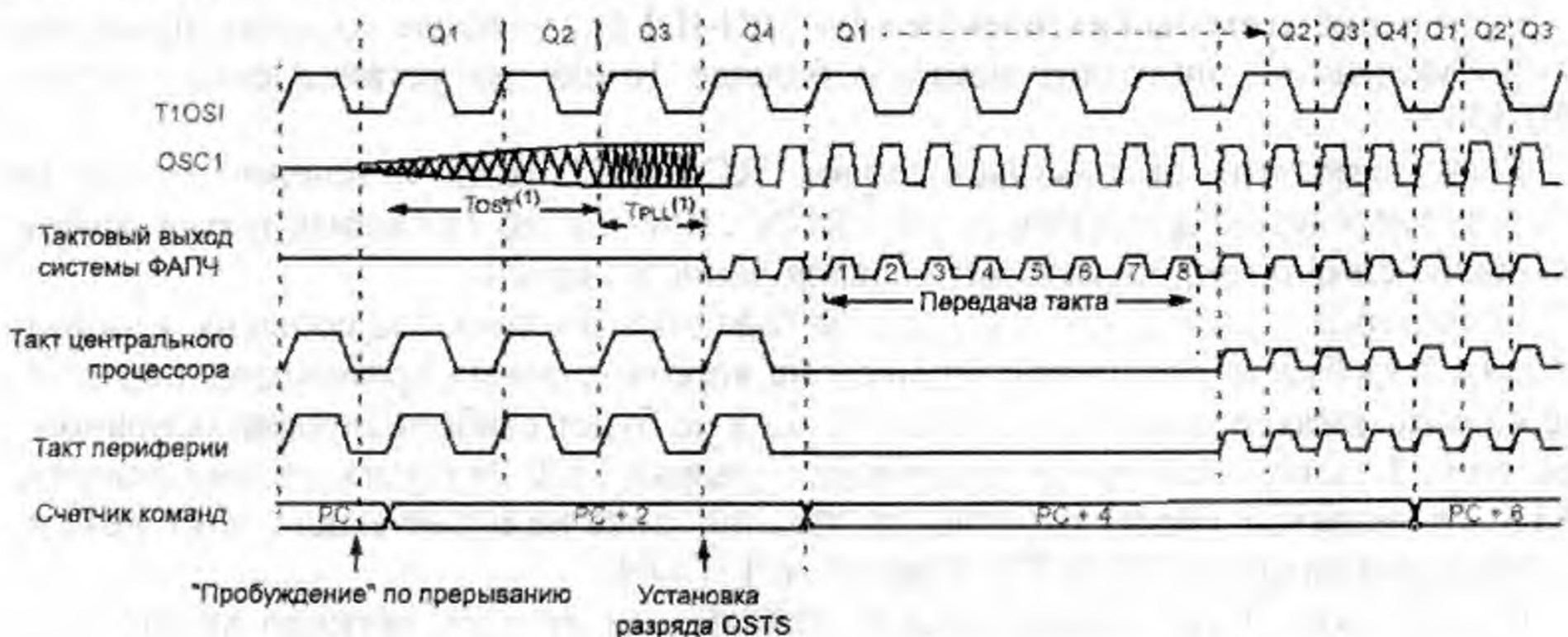
Рис. 4.2. "Пробуждение" из вспомогательного режима "RUN"
