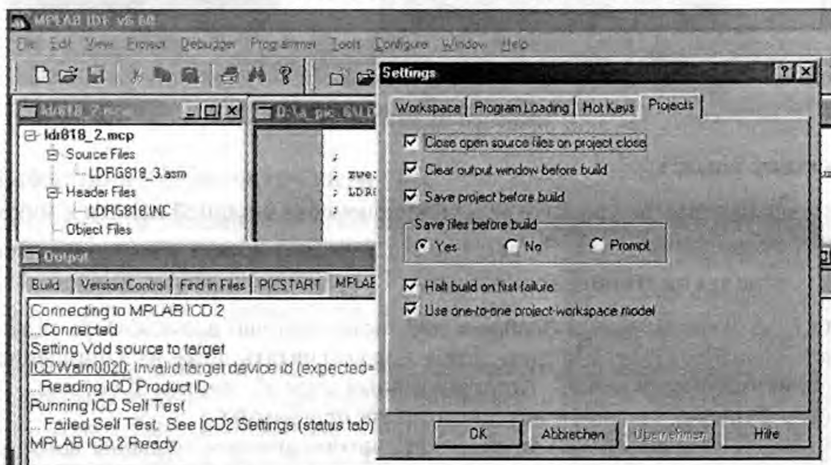
Рис. 8.23. Вкладка Projects диалогового окна Settings
