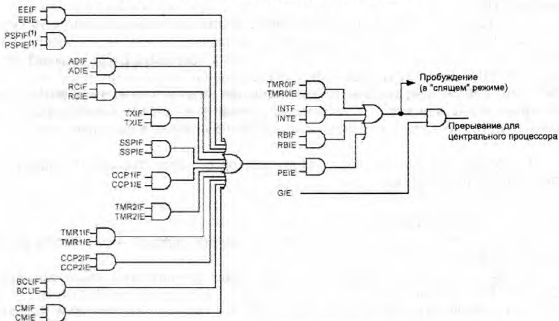
Рис. 3.2. Типичная структура прерываний PIC18
