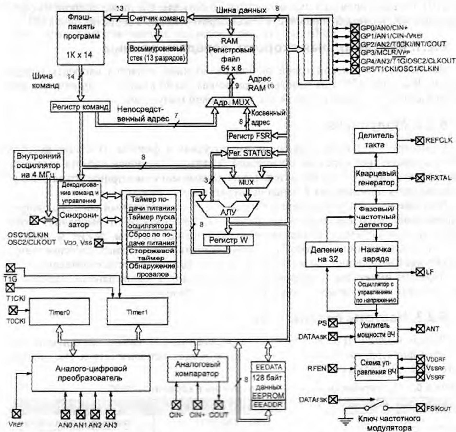
Рис. 6.1. Блок-схема микроконтроллера rfPIC
