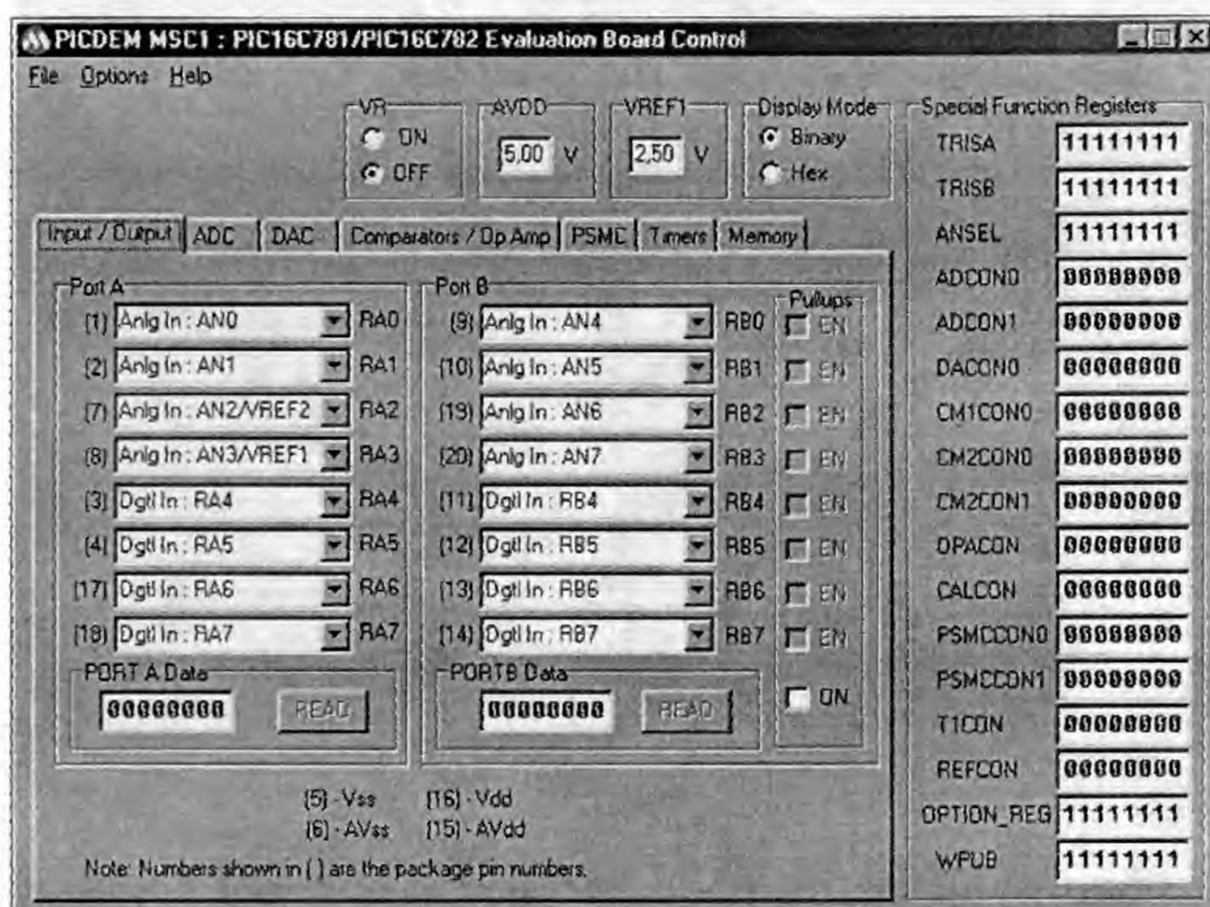
Рис. 10.17. Графический интерфейс набора PIC-MSC
