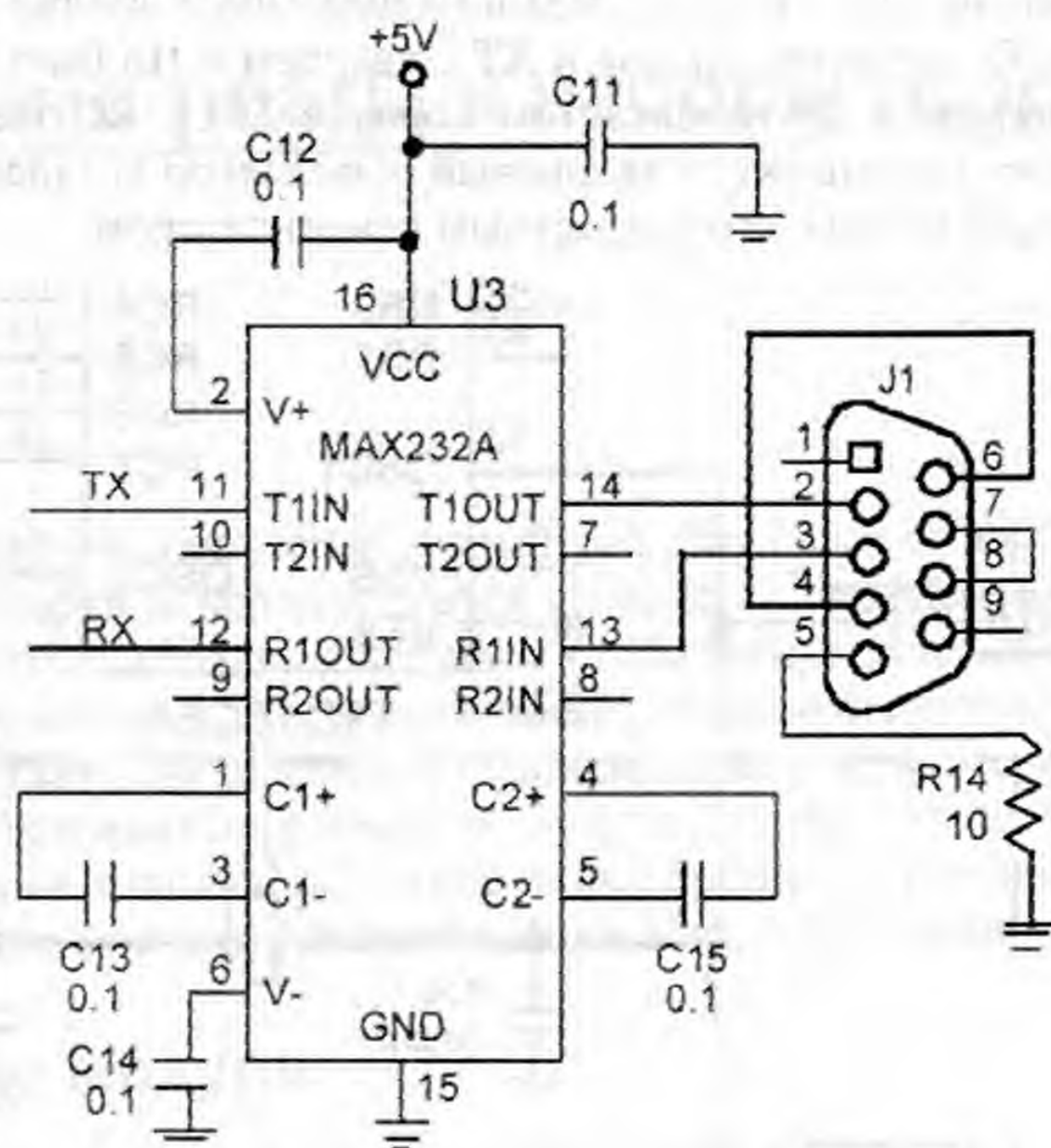
Рис. 10.3. Схема управления V.24 с девятиконтактным разъемом DSUB
