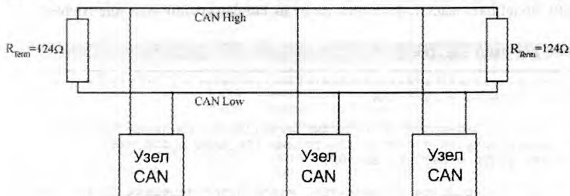
Рис. 2.2. Устройство сети CAN
