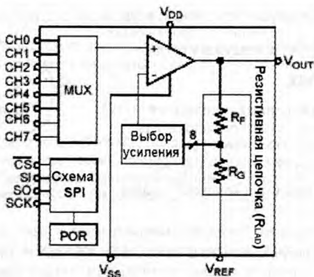
Рис. 11.12. PGA с восемью входными каналами
