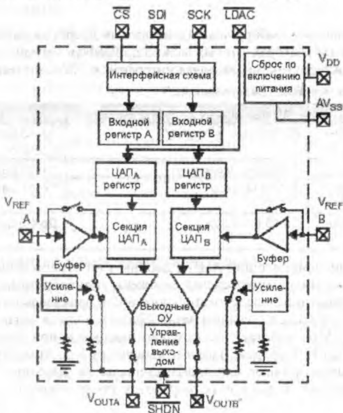
Рис. 11.16. ЦАП с двумя силовыми выходами (в MCP4921 — только один выход)
