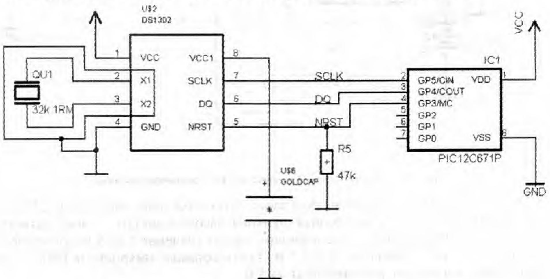
Рис. 11.30. Сопряжение микроконтроллера PIC и микросхемы DS1302
