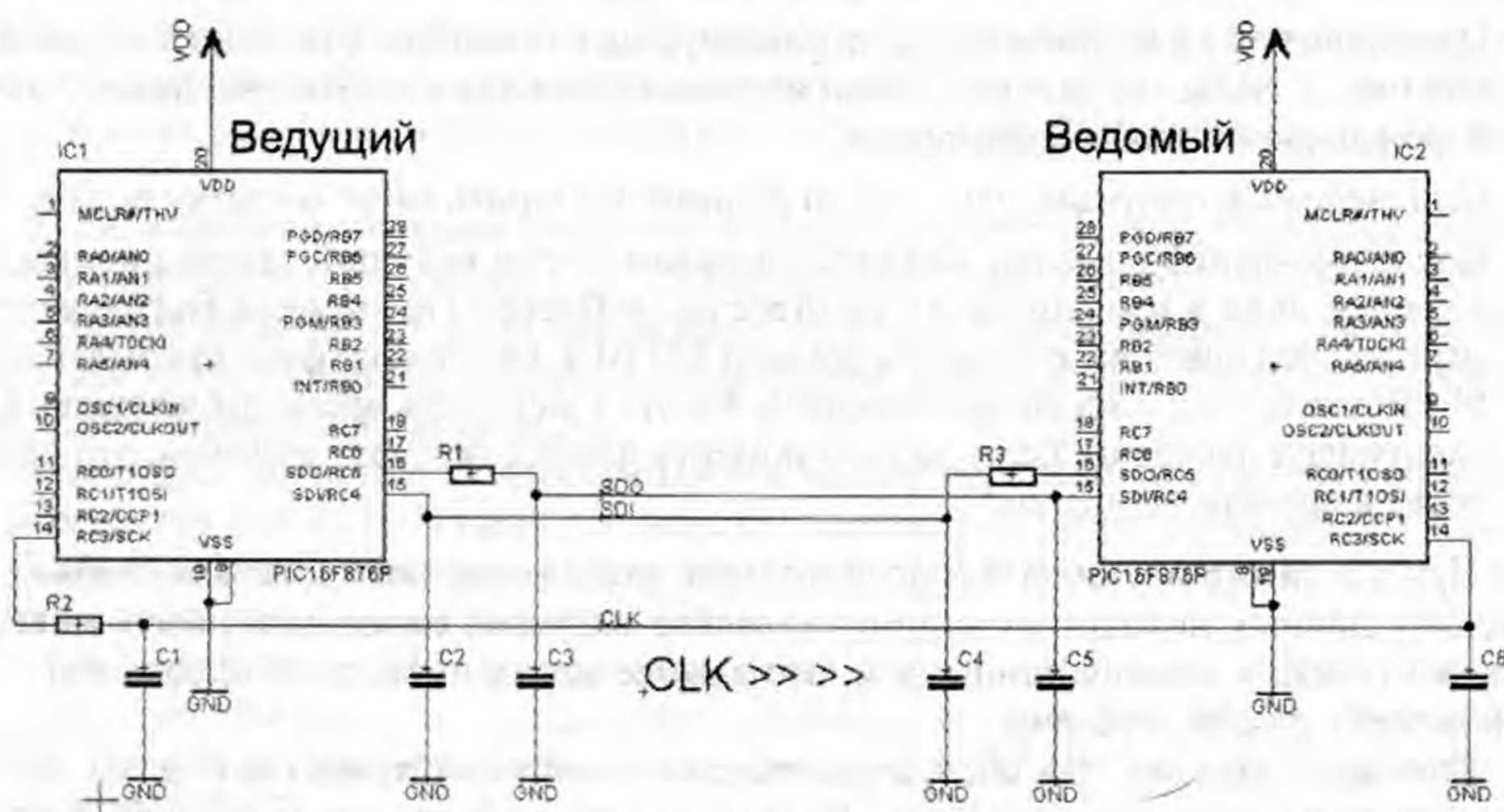
Рис. 2.1. Решение проблем с SPI
