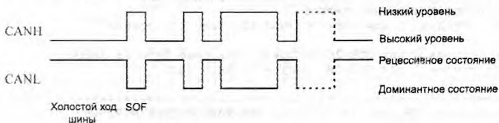
Рис. 2.3. Сигнал в шине CAN
