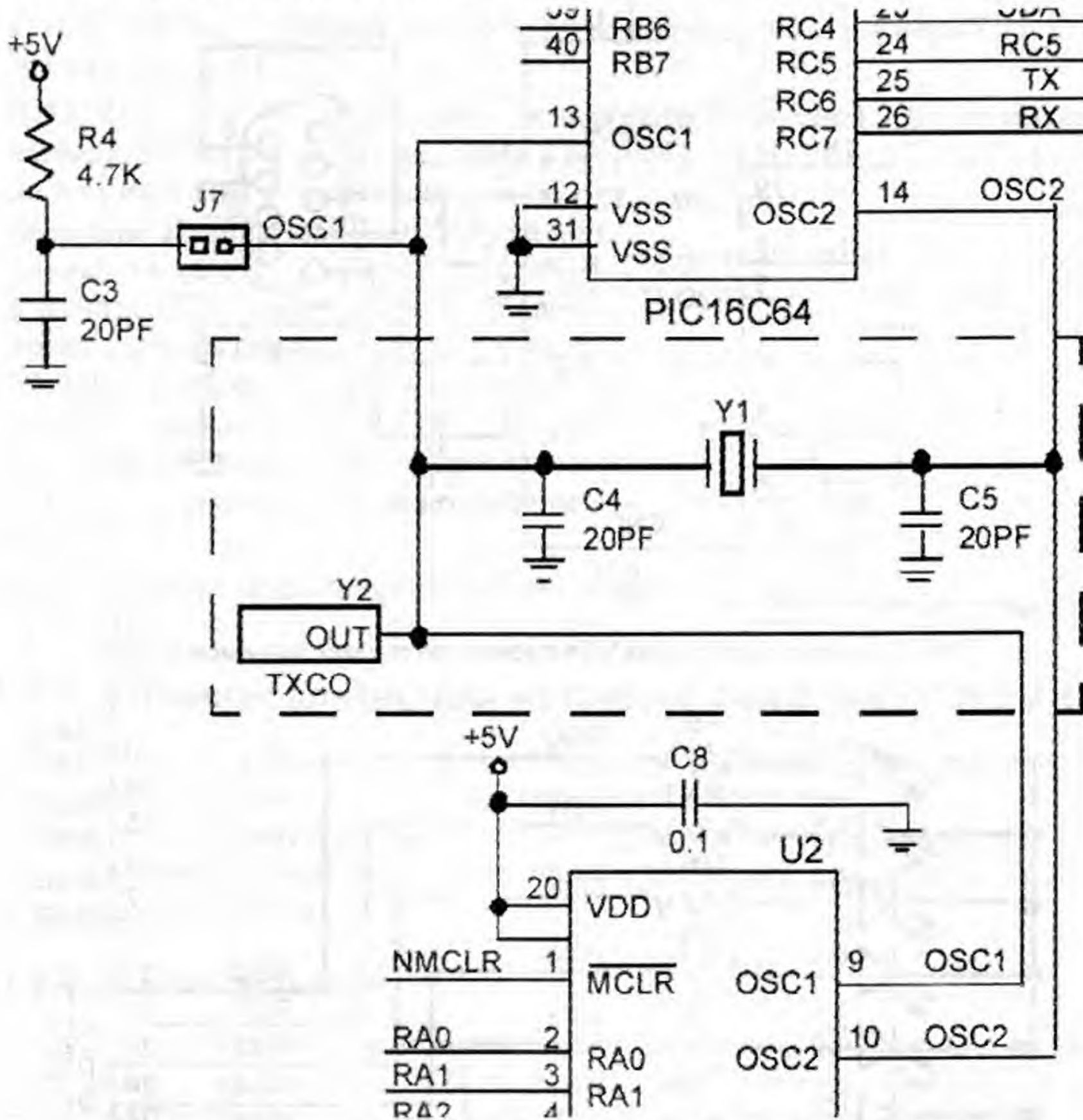
Рис. 10.2. Возможность подключения внешней схемы осциллятора
