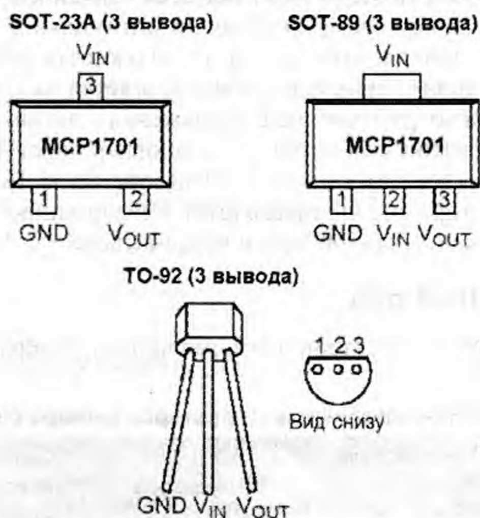
Рис. 11.22. Различные варианты корпуса для MCP1701
