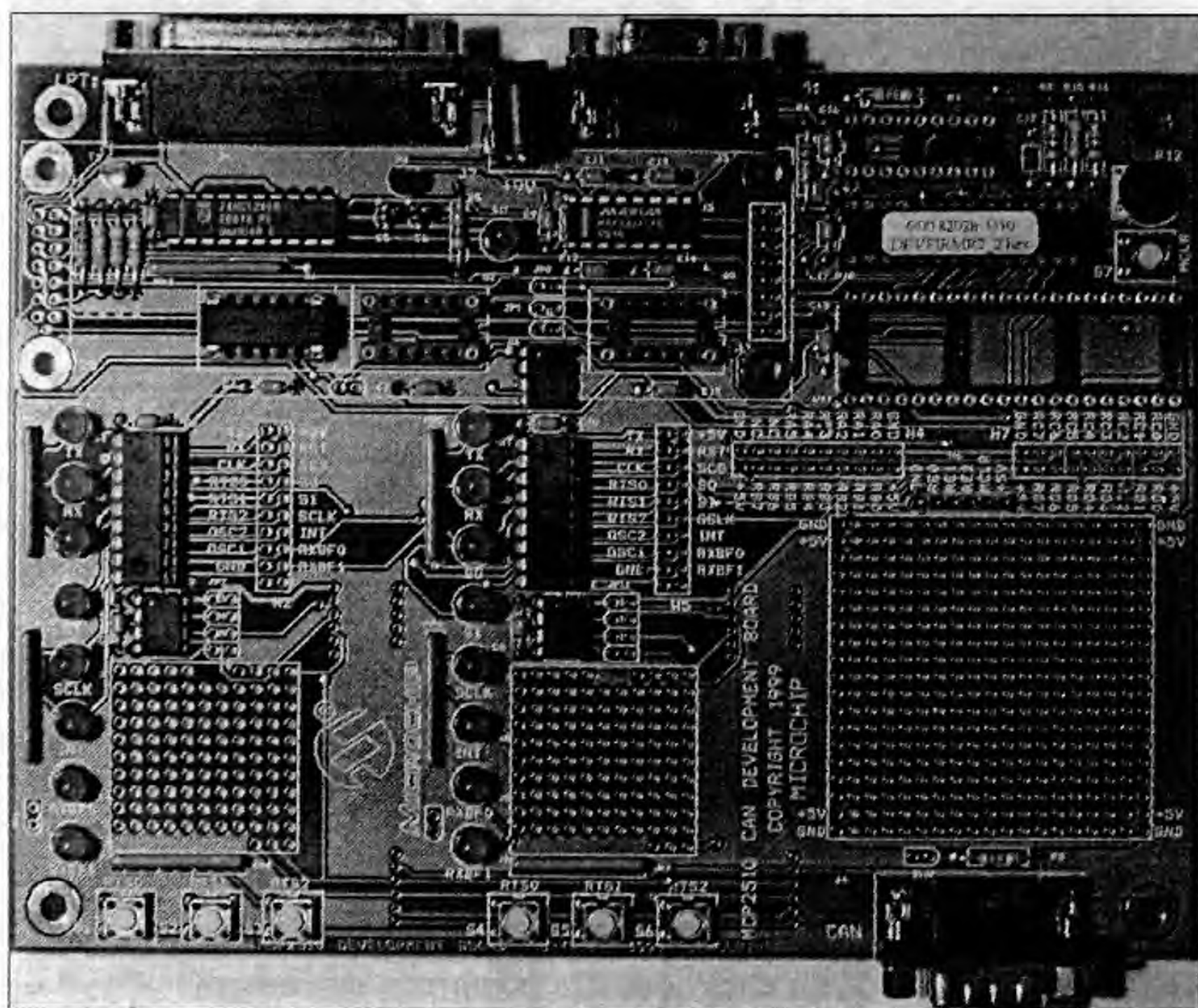
Рис. 10.18. Демо-плата MCP2510
