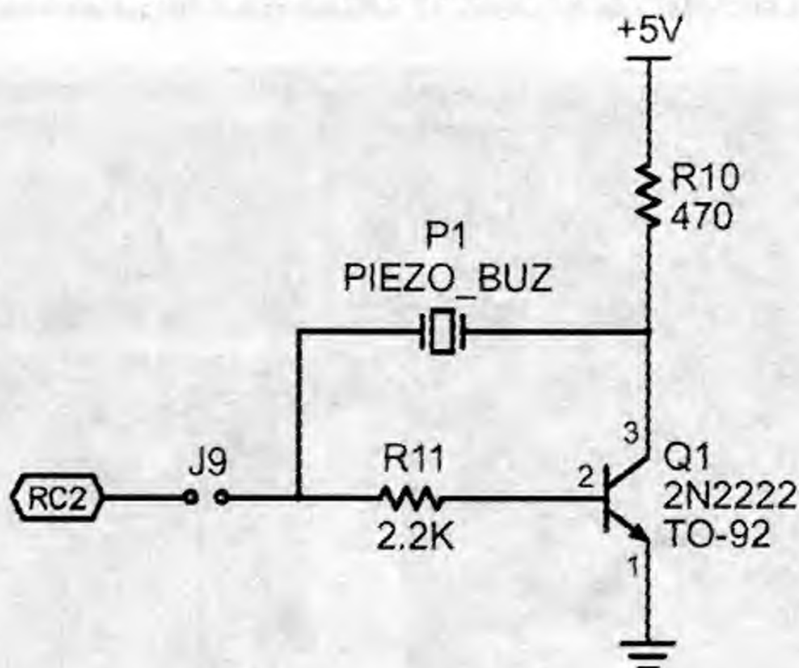
Рис. 10.9. Схема включения зуммера платы PICDEM2 plus
