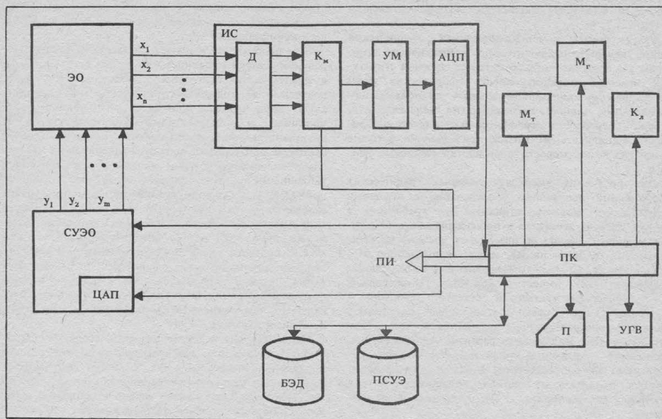
Рис. Типовая схема автоматизации экспериментальных исследований:
