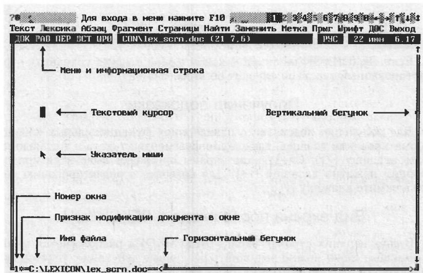
Рис. 28.1 Вид экрана после входа в ЛЕКСИКОН
