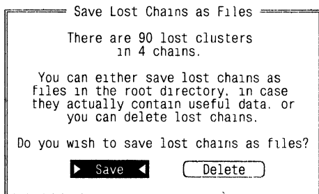
Рис. 10.6. Запрос о способе возврата «потерянных» участков на диске
