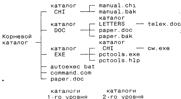
Рис 5.1. Пример файловой системы на магнитном диске
