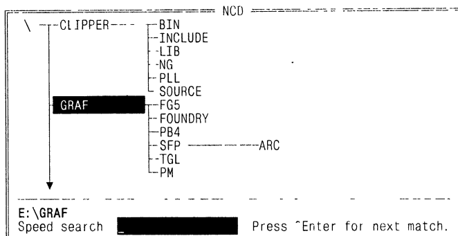
Рис. 15.1 Быстрый переход в другой каталог
