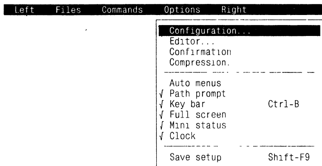
Рис. 16.4 Меню Norton Commander — пункт «Options»
