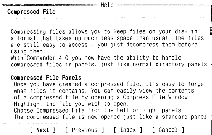
Рис. 12.2. Пример экрана помощи, выдаваемого при нажатии F1
