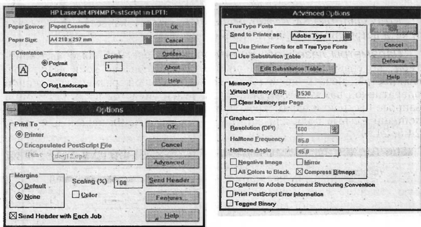
Рис. 24.7. Запросы параметров драйвера принтера HP LaserJet 4MP (запрос слева сверху — головной, запрос слева внизу вызывается из него нажатием кнопки Options (Параметры), а запрос справа — из запроса слева внизу нажатием кнопки Advanced (Дополнительно))
