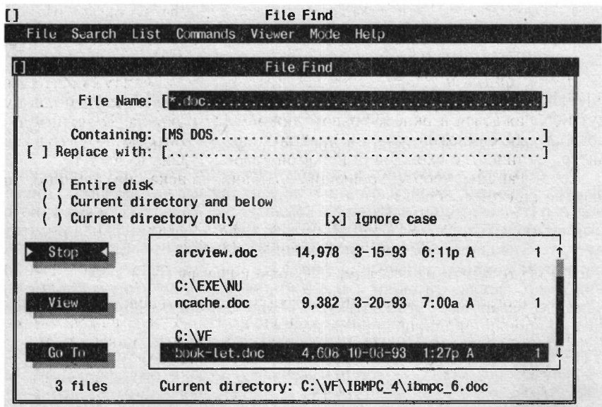
Рис. 7.1 Экран со списком файлов, найденных программой FileFind
