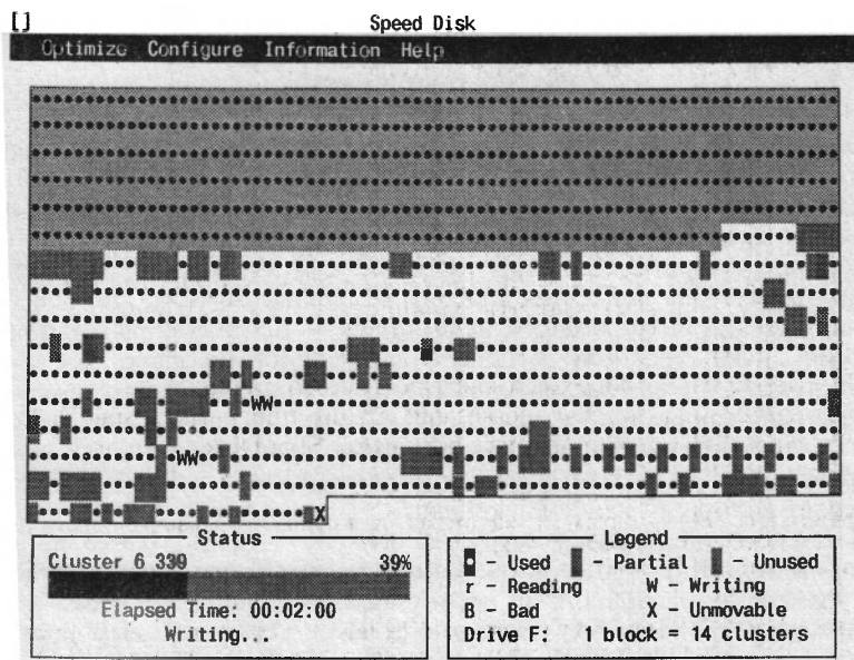
Рис. 10.9. Сжатие диска программой SpeedDisk
