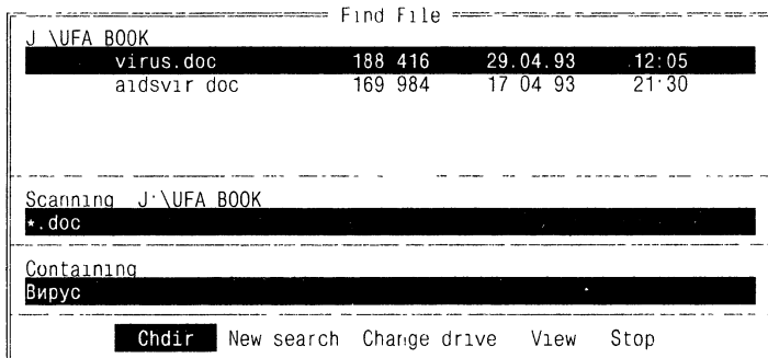
Рис. 14.3. Быстрый поиск файла на диске
