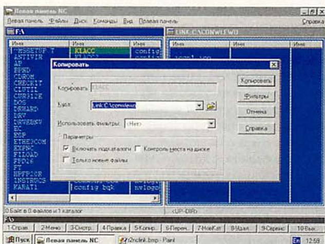
Копирование каталога KLACC с диска F: «ведущего» ПК в каталог C:\CONWLEW «ведомого»
