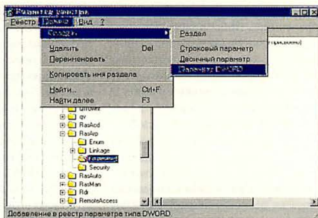
Включение внутреннего маршрутизатора Windows NT
