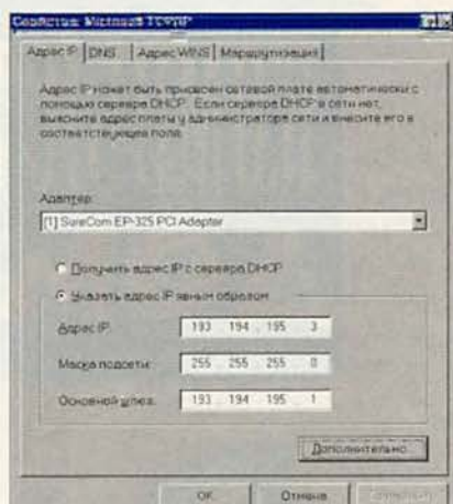
Установка TCP/IP-адресов в Windows NT
