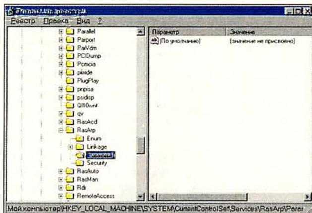
Задание параметра в реестре Windows NT
