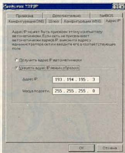
Установка TCP/IP-адресов в Windows 95
