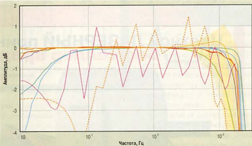
Рис.С. Результаты измерений АЧХ записи
