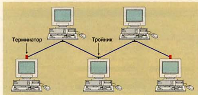
Подключение коаксиального кабеля
