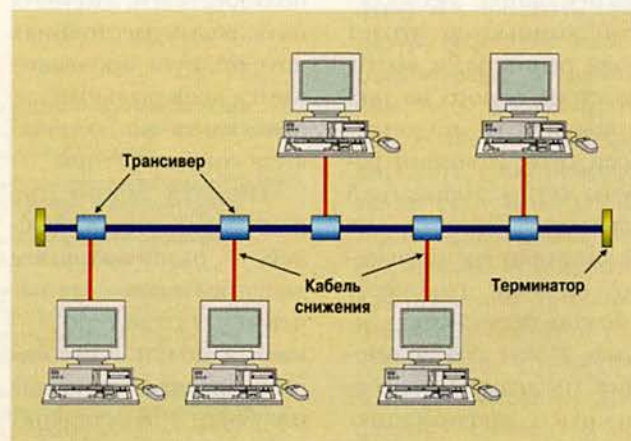
Магистраль на толстом коаксиальном кабеле
