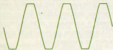
Вид искаженного сигнала при ограничении по «насыщению» (входной сигнал — синусоида)
