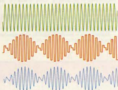
Рис. А. Биения выходного сигнала
