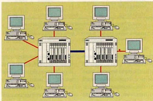
Сеть с топологией «звезда-шина»
