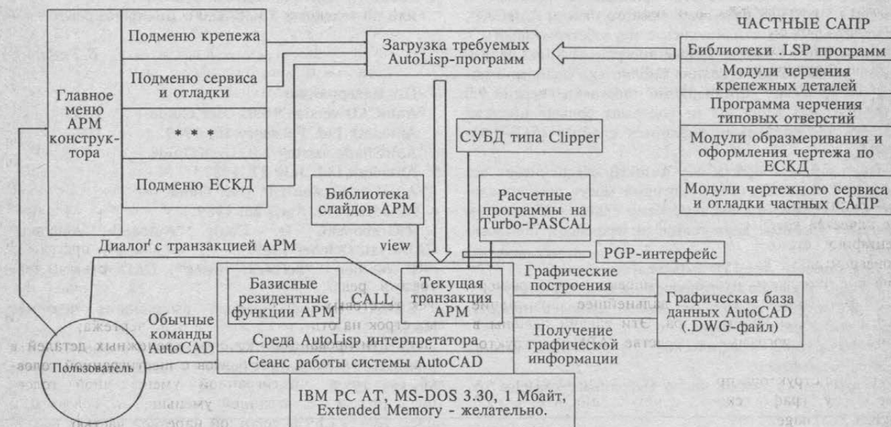
Рис.1. Функциональная схема АРМ конструктора.
