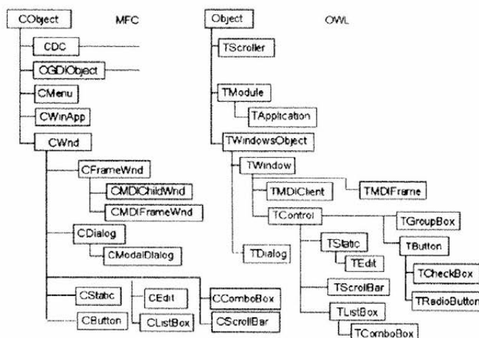
Иерархия классов MFC и OWL
