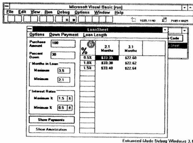
Рис. 1. Visual Basic 3.0
