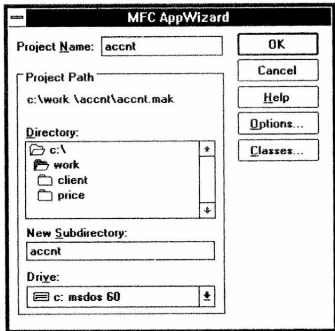
Рис. 1. Программа AppWizard
