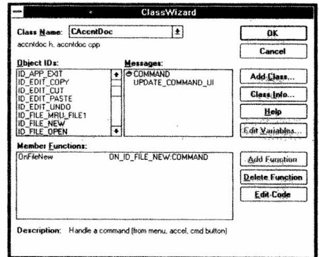
Рис. 6. Программа ClassWizard
