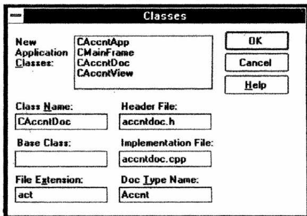
Рис. 3. Задание имен классов
