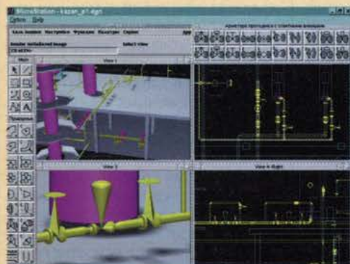
Фрагмент установки для подготовки пирогаза на АО «Казаньоргсинтез». OMNI-Series. Русская версия
